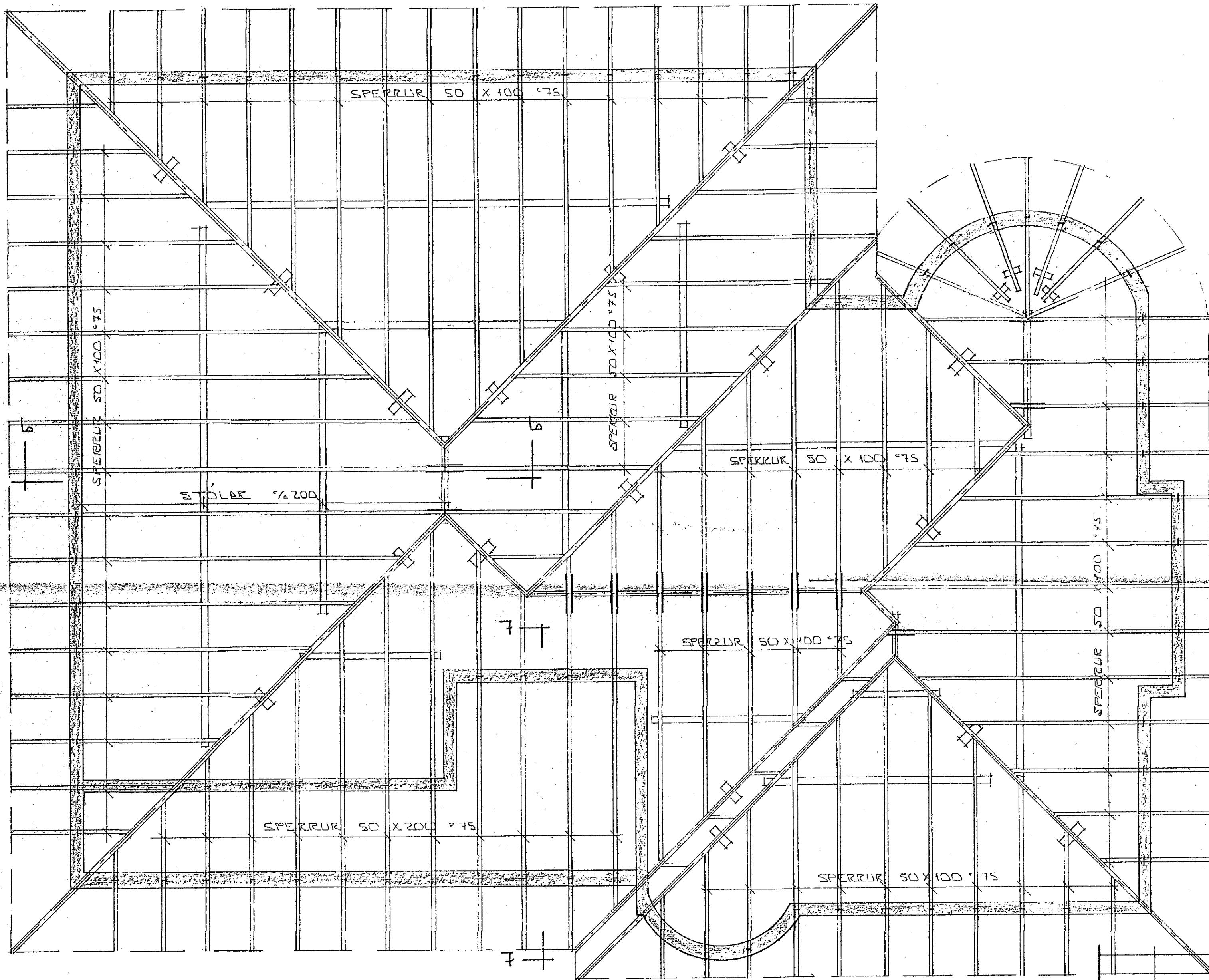
GRUNNMYND 1:50
