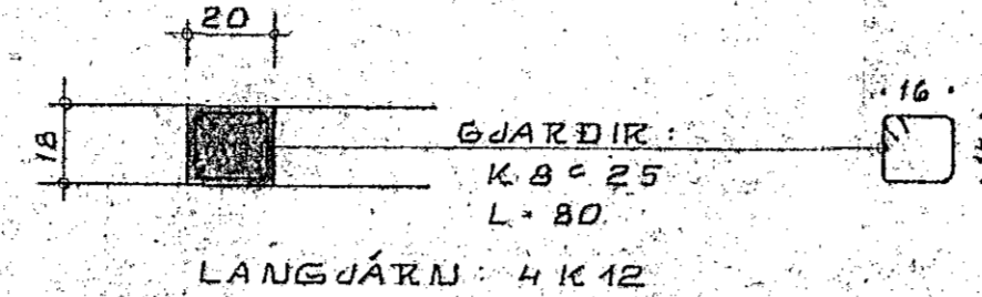
SÚLA S.2 1:20
