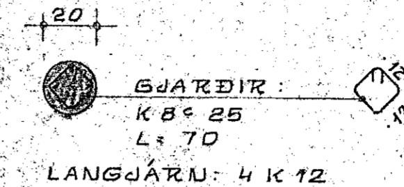
SÚLA S.3 1:20
