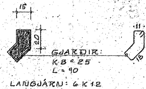
SÚLA S.5 1:20
