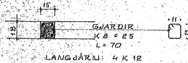
SÚLA S.1 1:20
