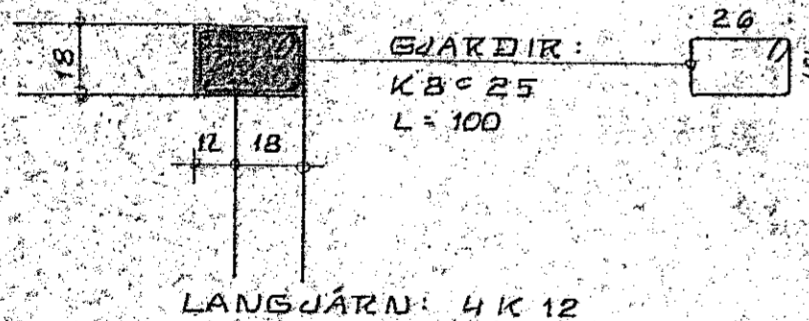
SÚLA S.7 1:20
