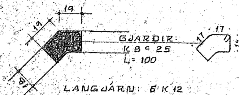
SÚLA S.4 1:20
