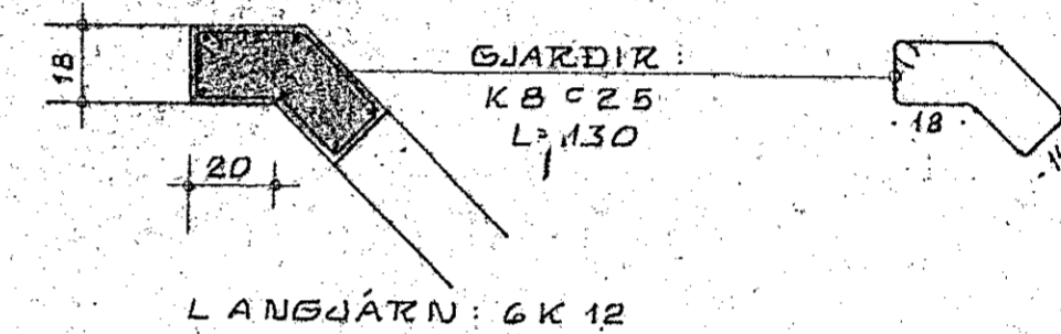
SÚLA S.6 1:20
