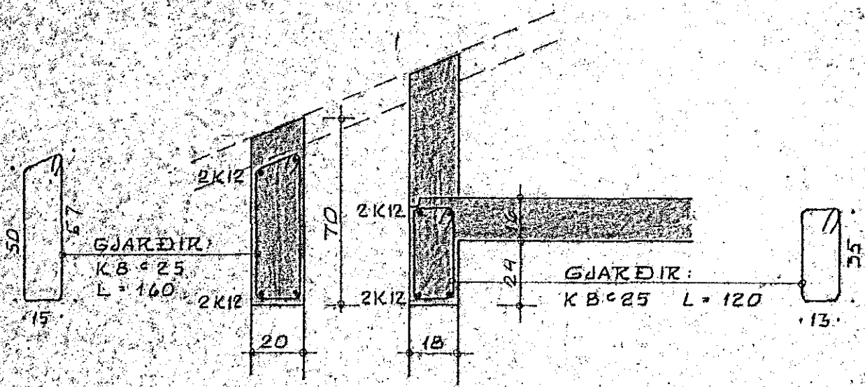
SNID 1-1 1:20
