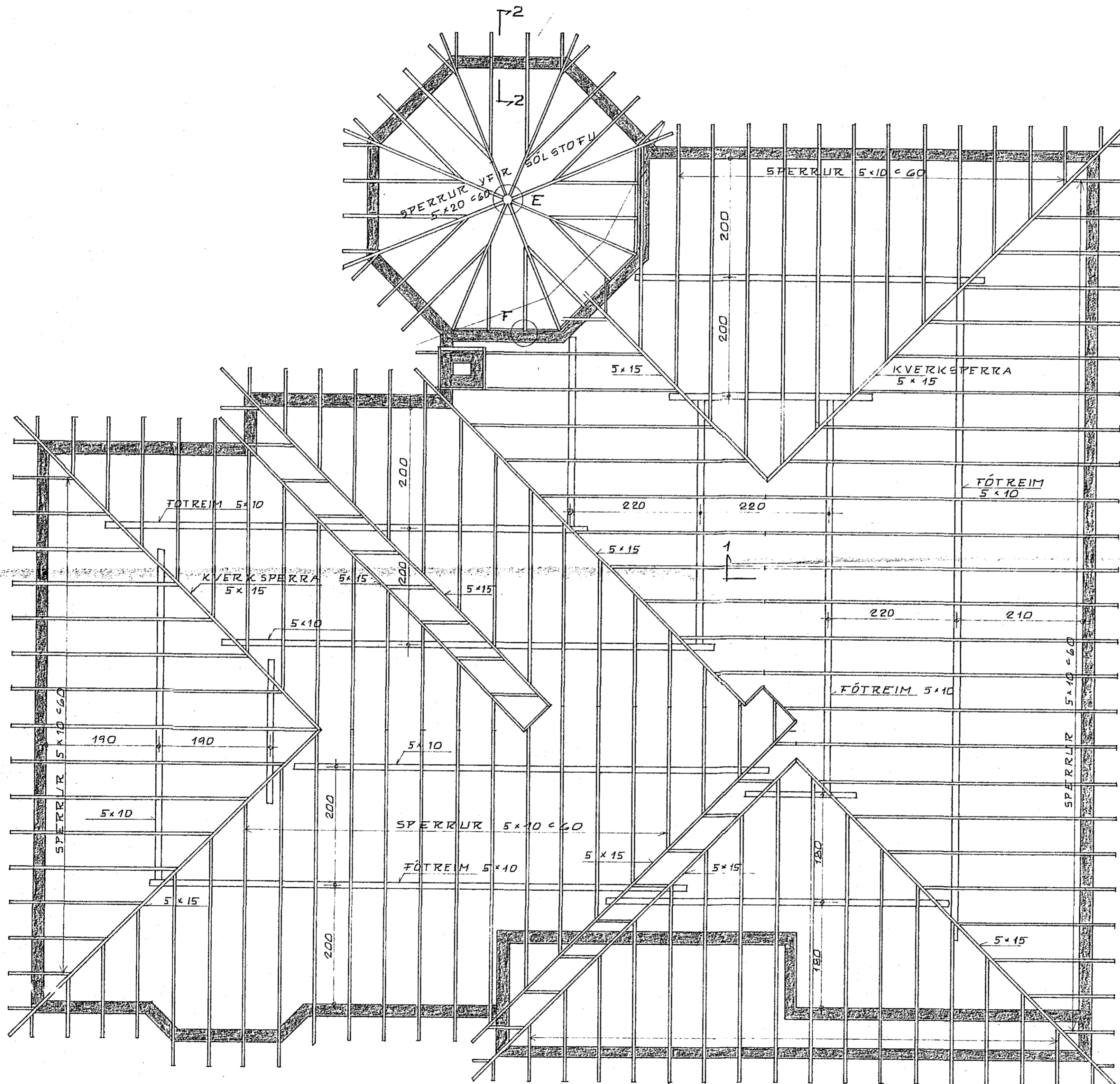
GRUNNMYND 1:50
