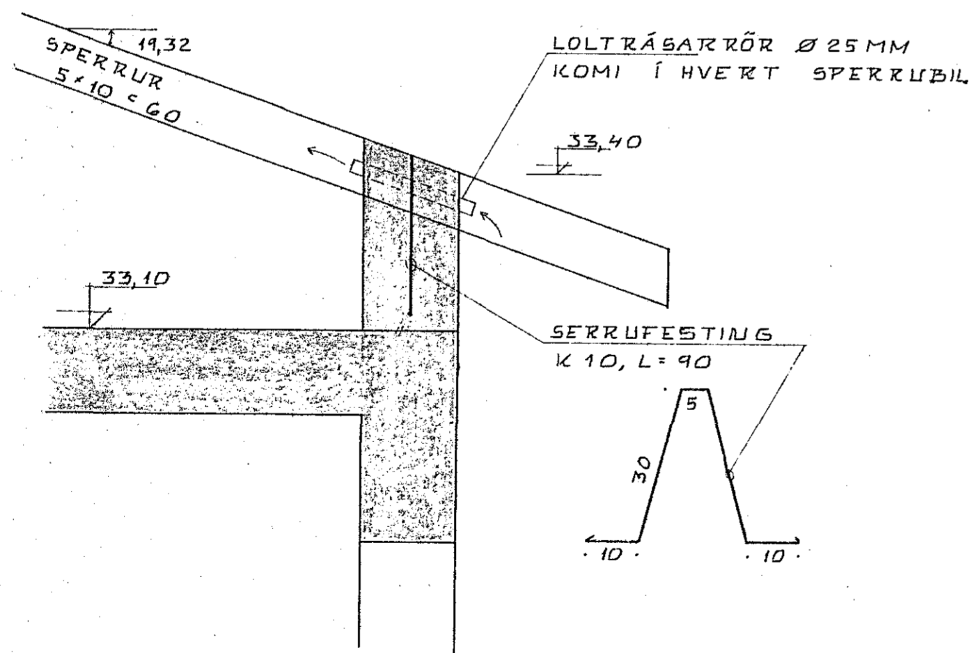
SÉRMYND C 1:10
