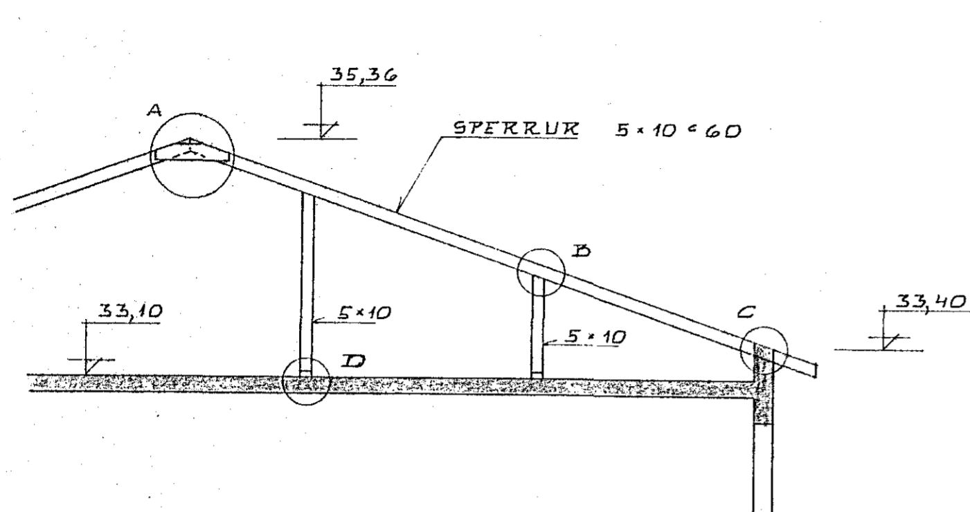
SNID 1:1 1:50
