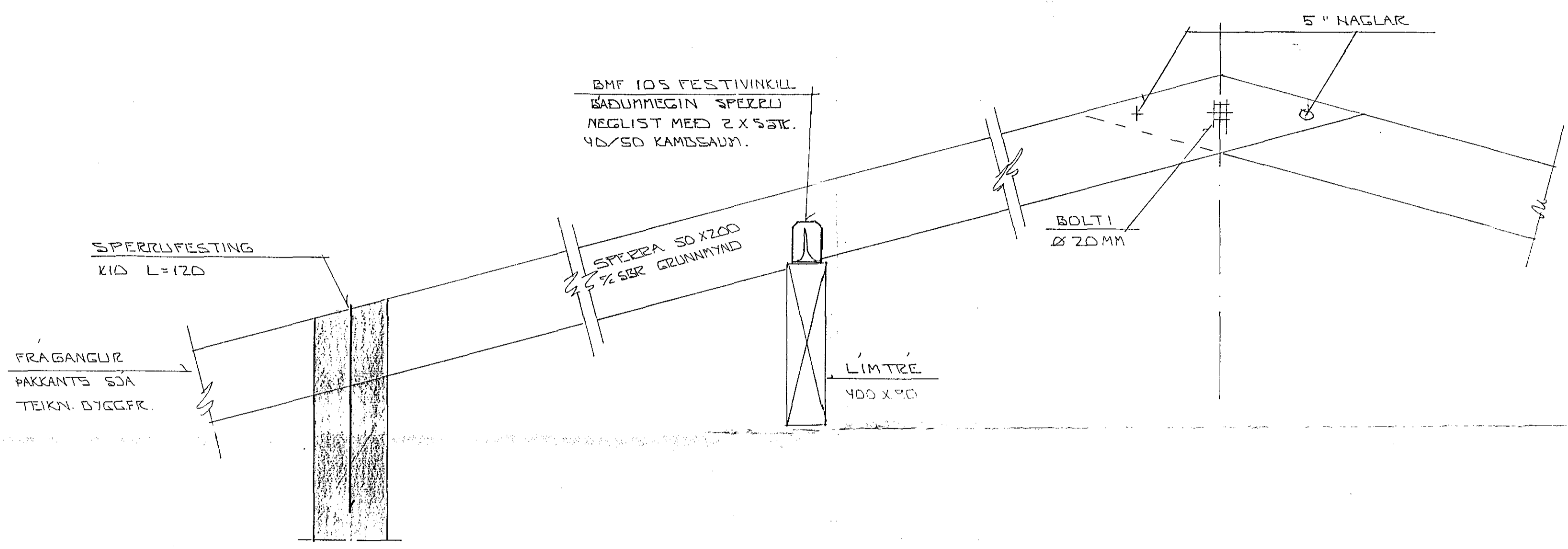
SNID 8 - 8 ~ 1:10
