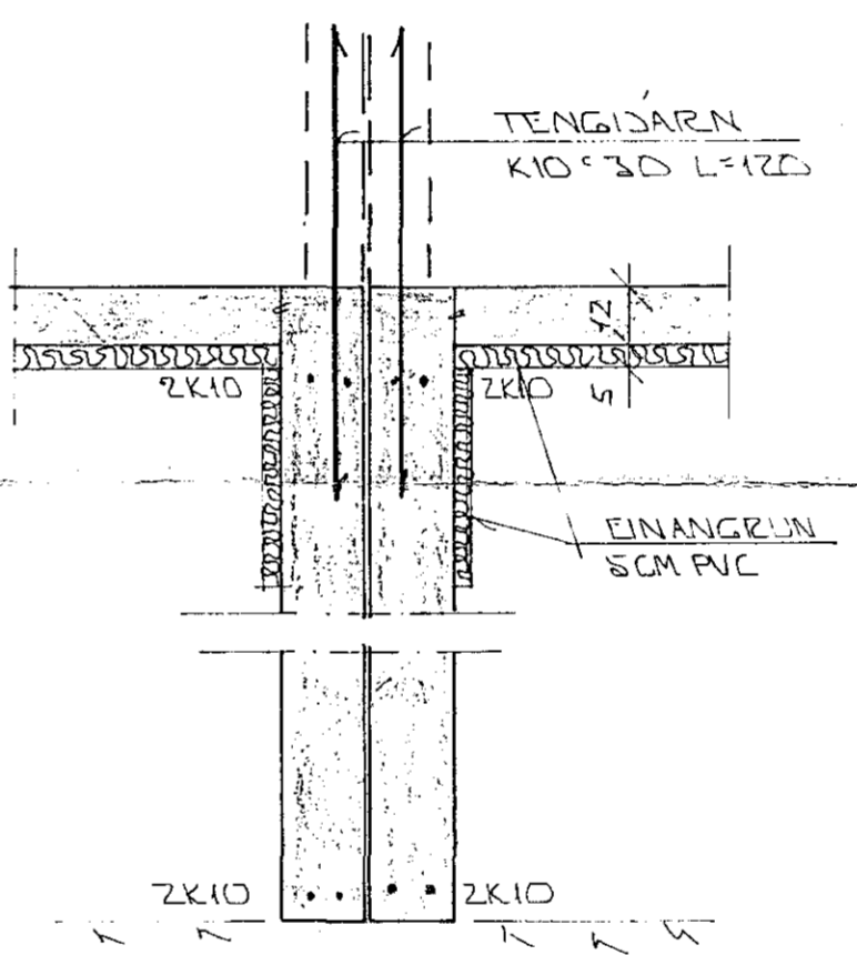
SNID 3 · 1:20
