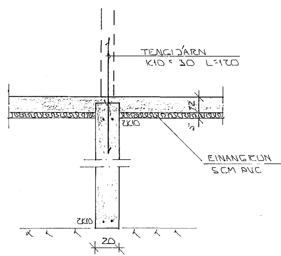
SNID 2 · 1:20
