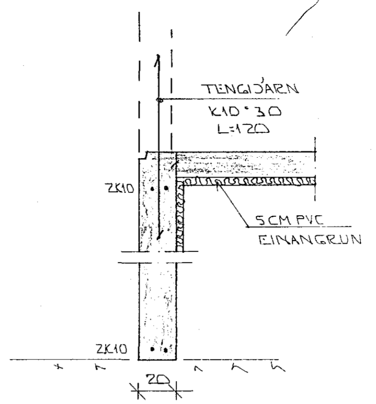
SNID 1 · 1:20
