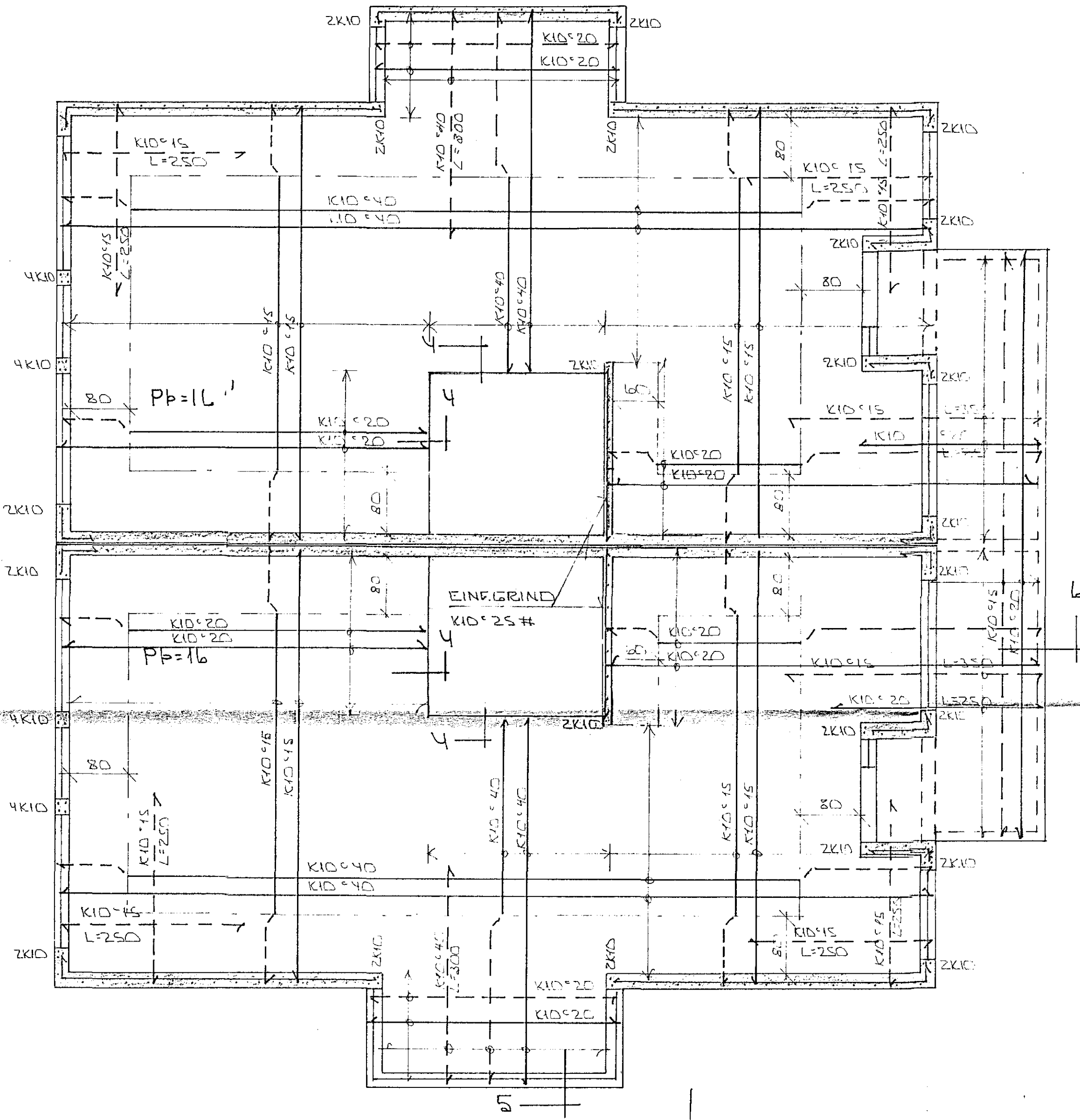
GRUNNMÝND 1:50
