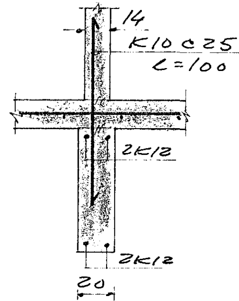
SNID B-B 1:20
