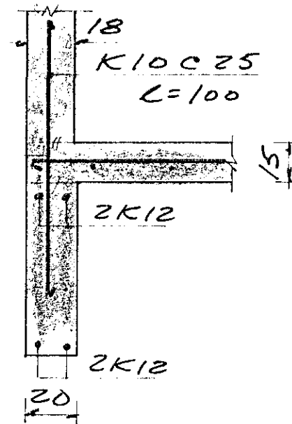
SNID A-A 1:20
