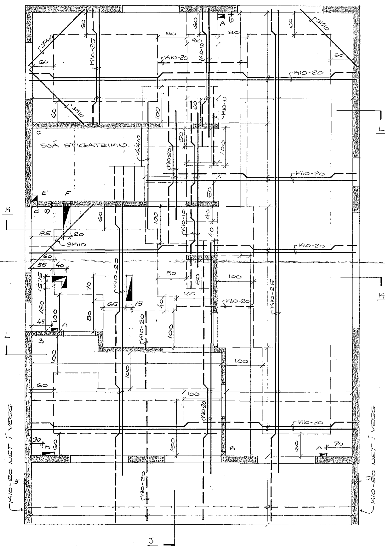
GRUNNMÁLND, M=1:80
