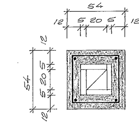
SKURÐUR A-A, M=1:20
