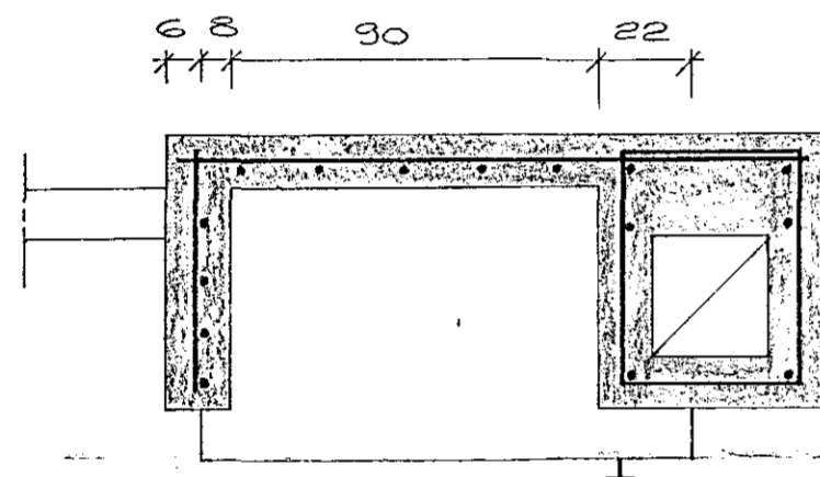
SKURÐUR C-C, M=1:20
