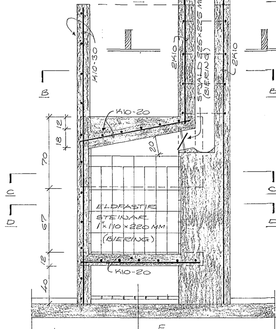
SKURÐUR F-F, M=1:20
