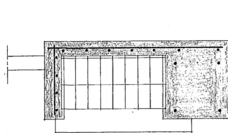
SKURÐUR D-D, M=1:20
