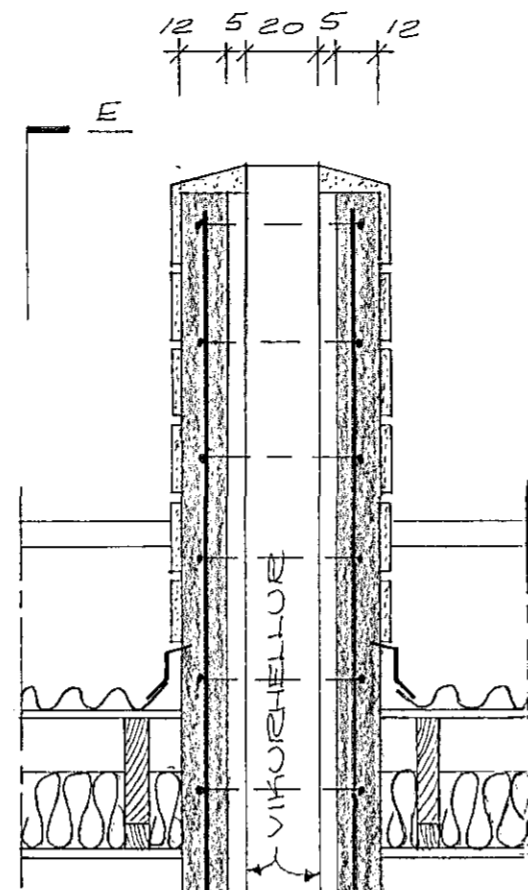
SKURÐUR A-A, M=1:20
