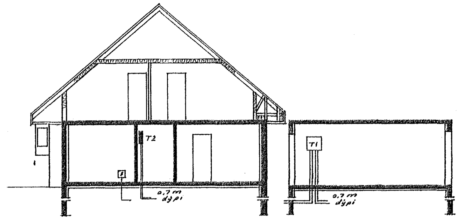
SNID A-A 1:100
