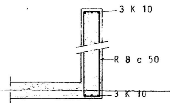
SNID D 1:20
