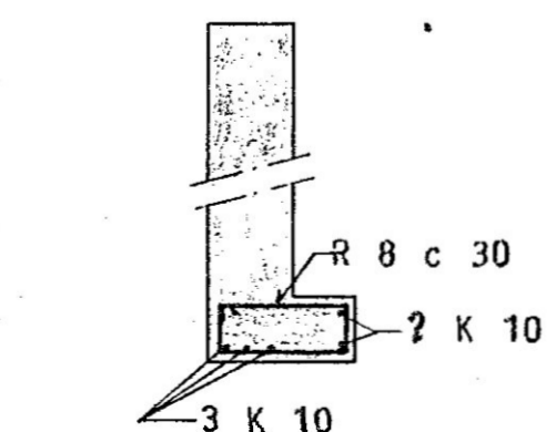
SNID G 1:20
