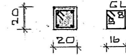
SULA S.1.1 1:20
