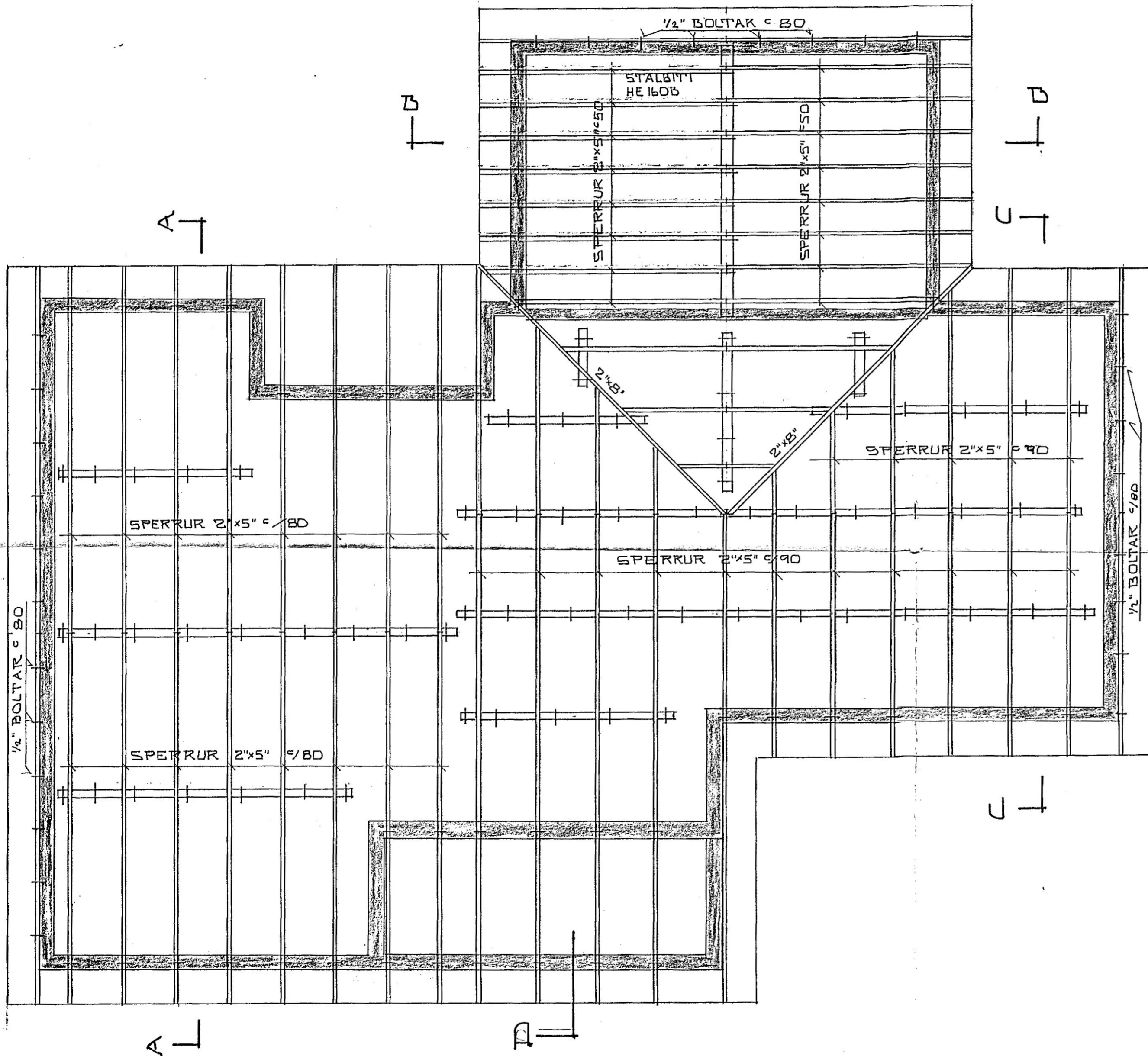
GRUNNMYND ÞAKS 1:50
