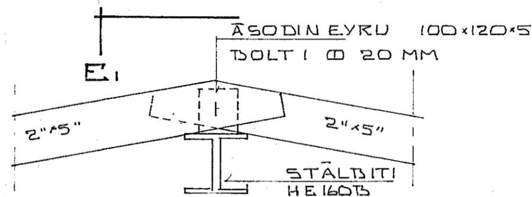
SERMYND E 1:10
