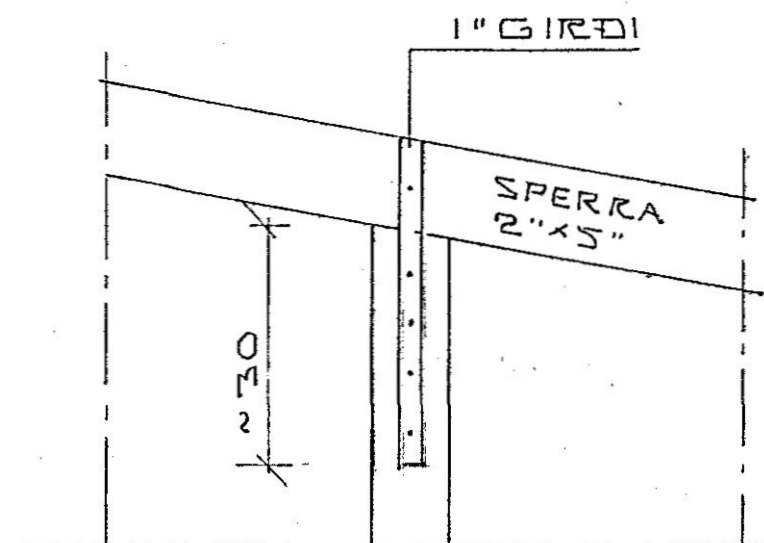
SERMYND B 1:10
