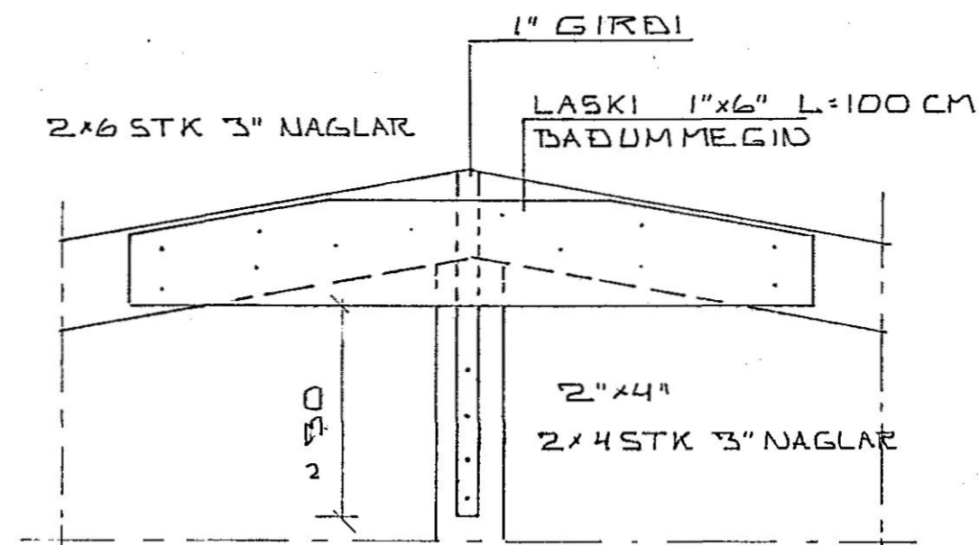
SERMYND A 1:10
