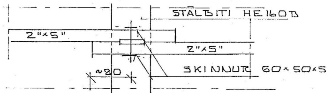
SNID E, 1:10
