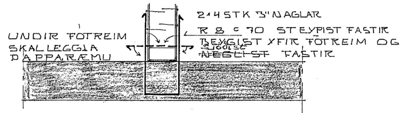
SERMYND D 1:10
