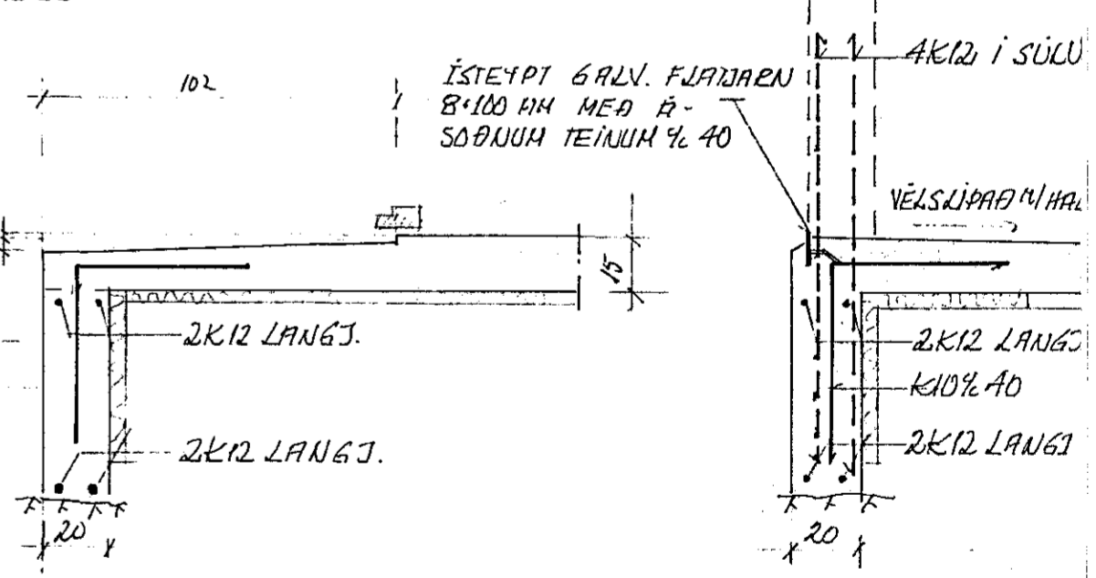
SNID E, 1:20
