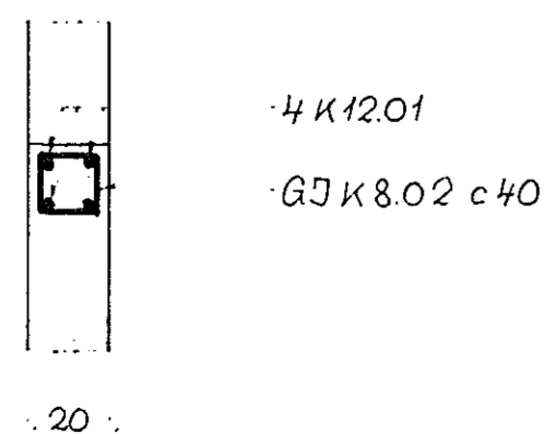
SNID Í S1.4. 1:20 2.stk.
