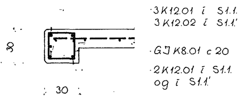
SNID Í S1.4. 1:20 2.stk.
