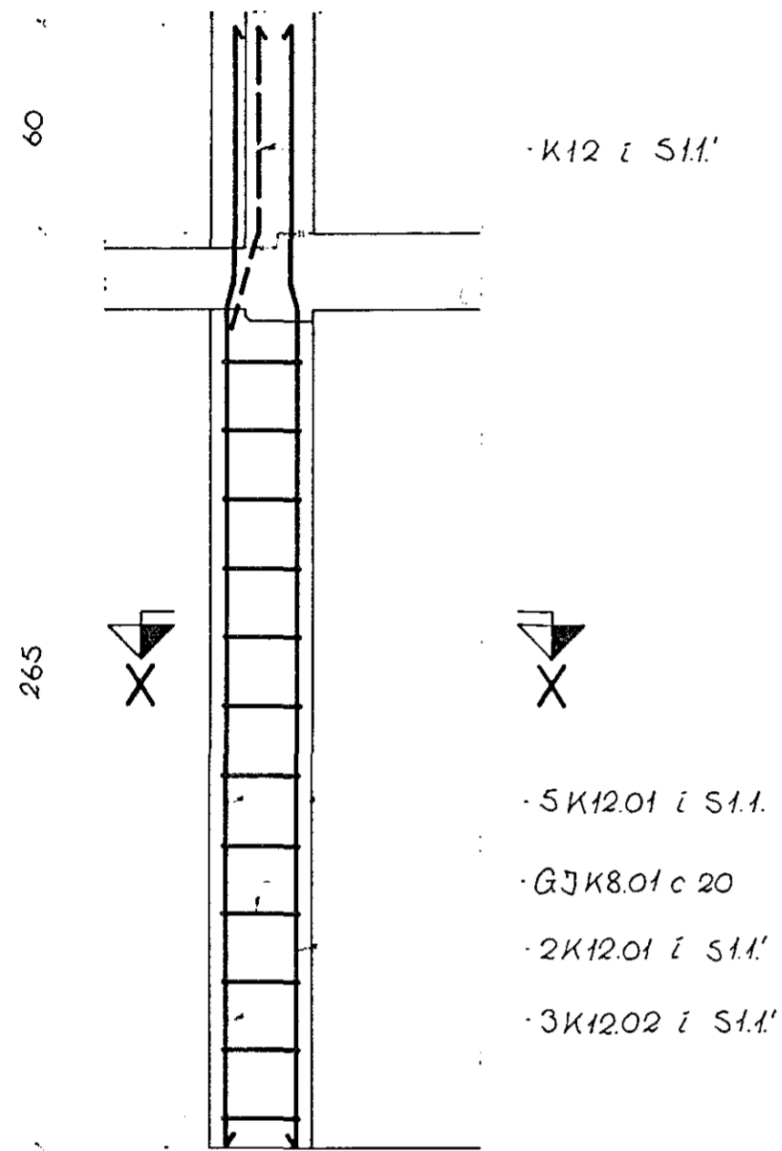
SÚLA S1.1. 1:20 1.stk. S1.1. 1.stk.
