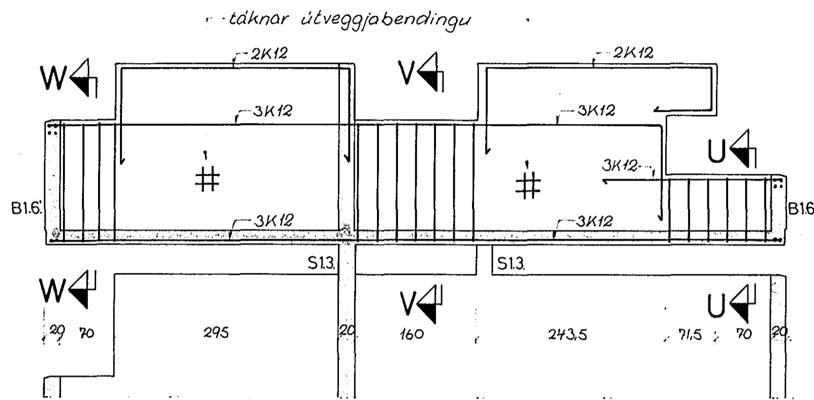
BITI B15. 1:50 1.stk.
