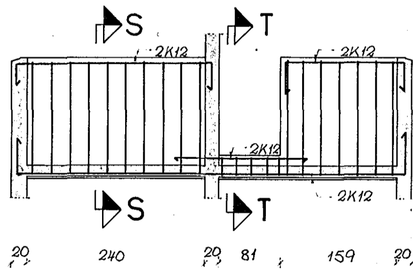
BITI B17. 1:50 1.stk.
