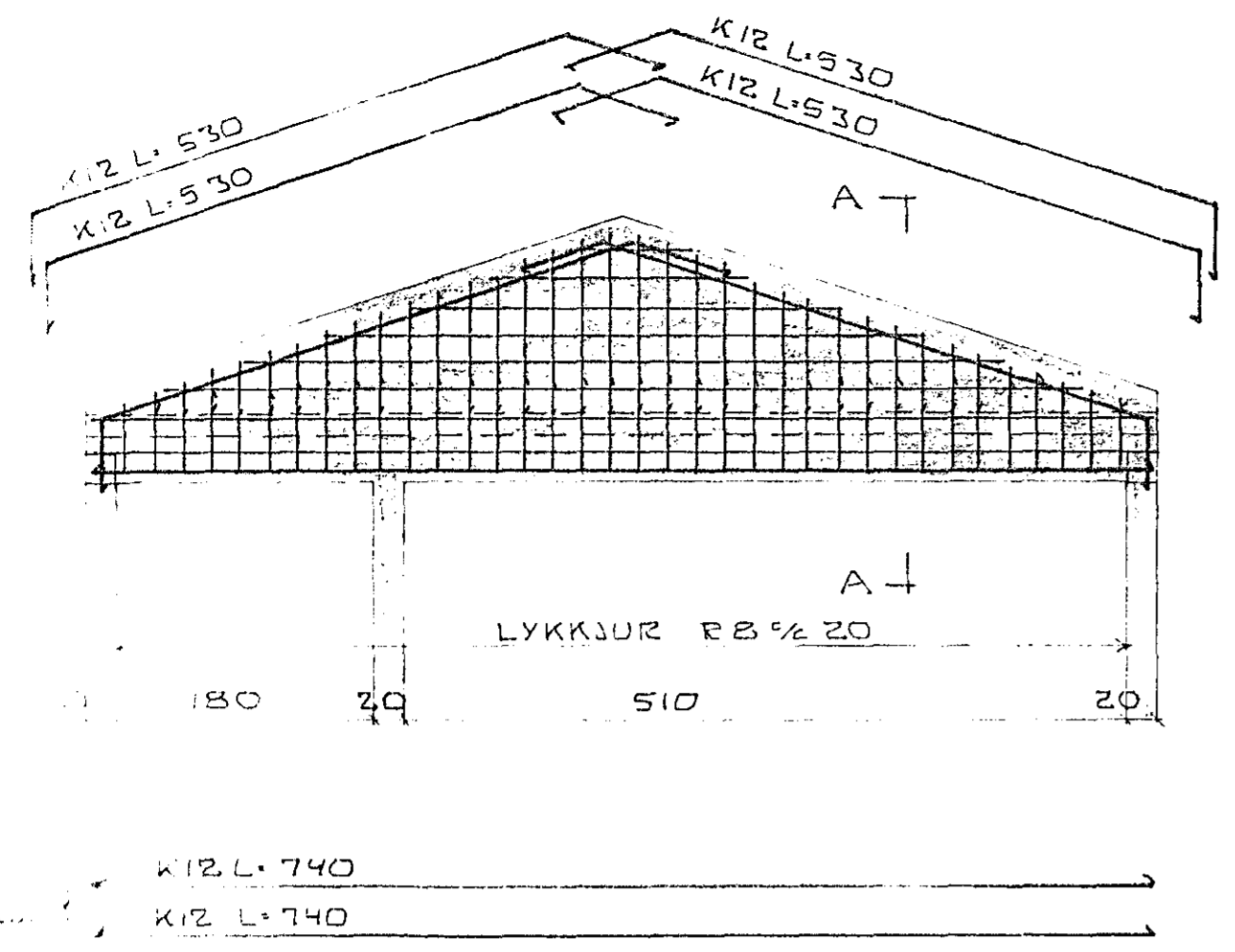
BITI B.1.1 1:50
