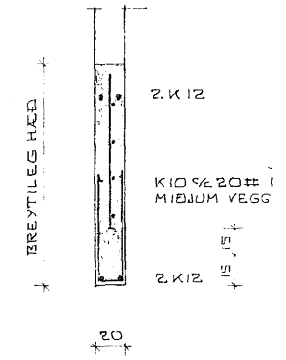
SNID A-A 1:20
