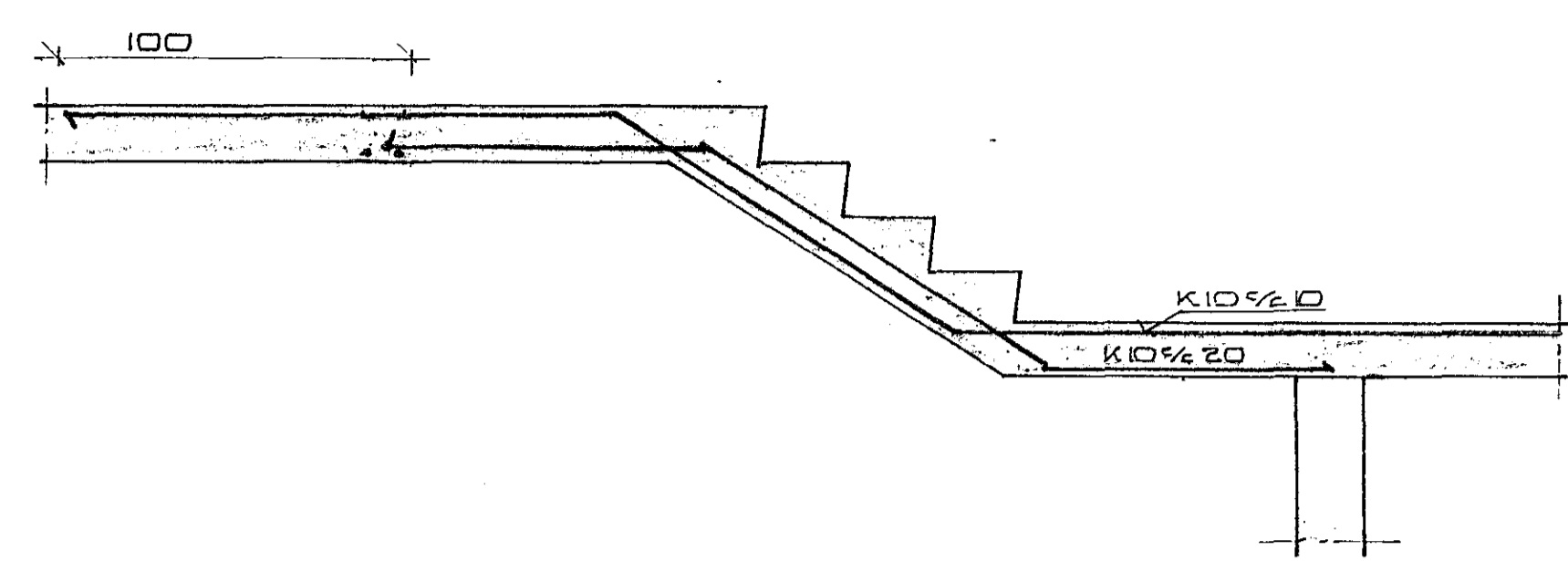
SNID A-A 1:20
