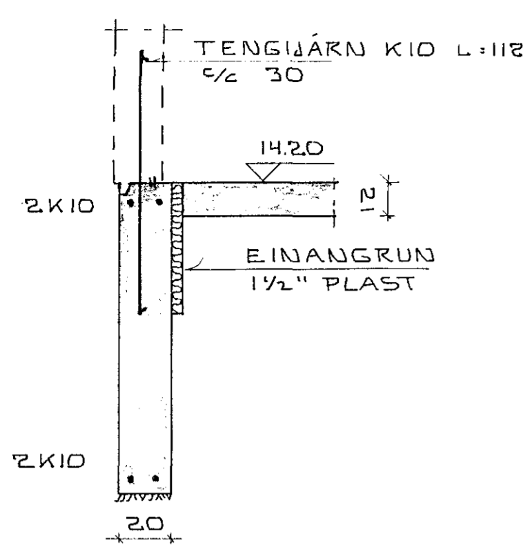
SNID A-A
