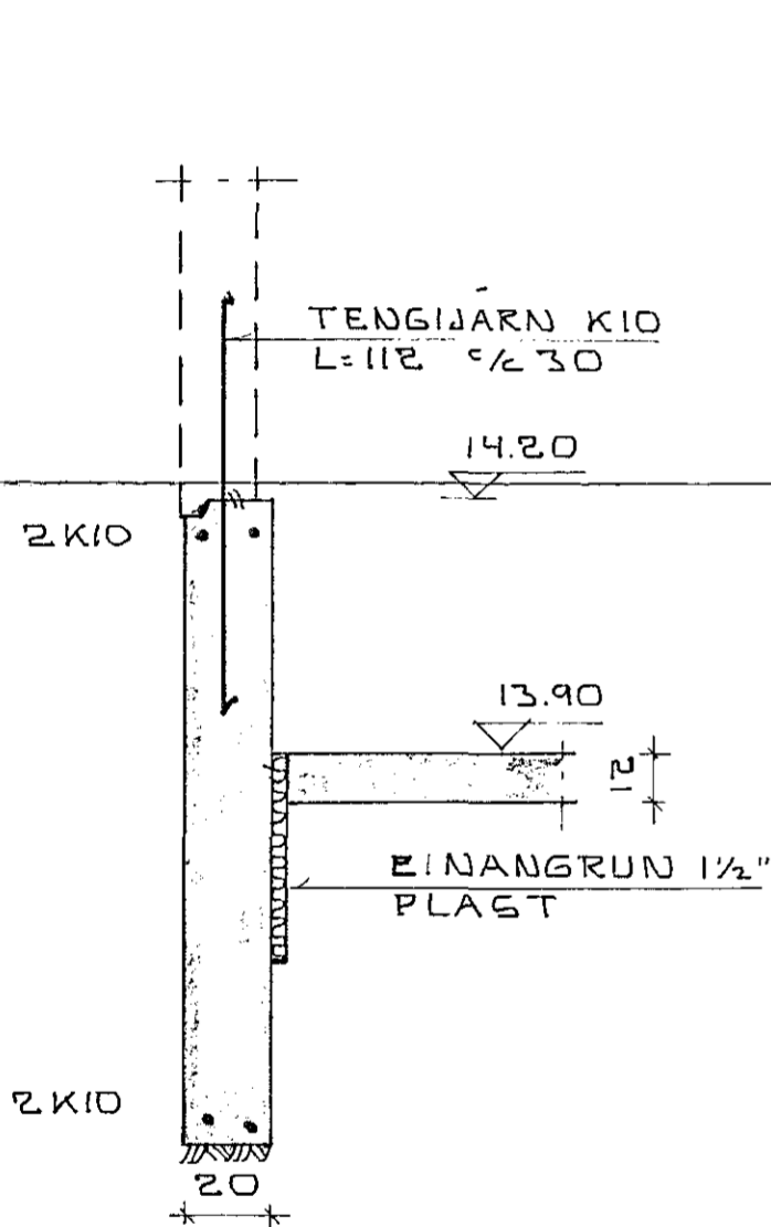
SNID A-A
