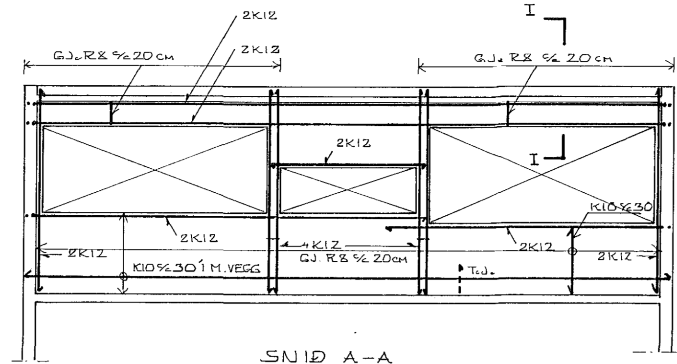
SNID A-A
