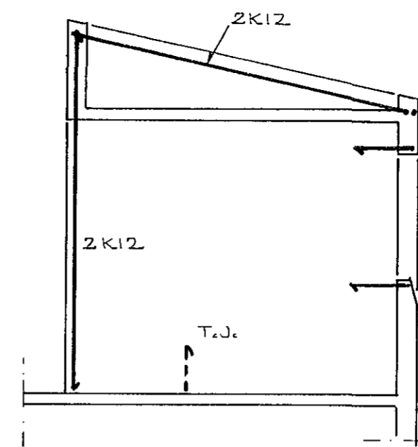
SNID D-D
