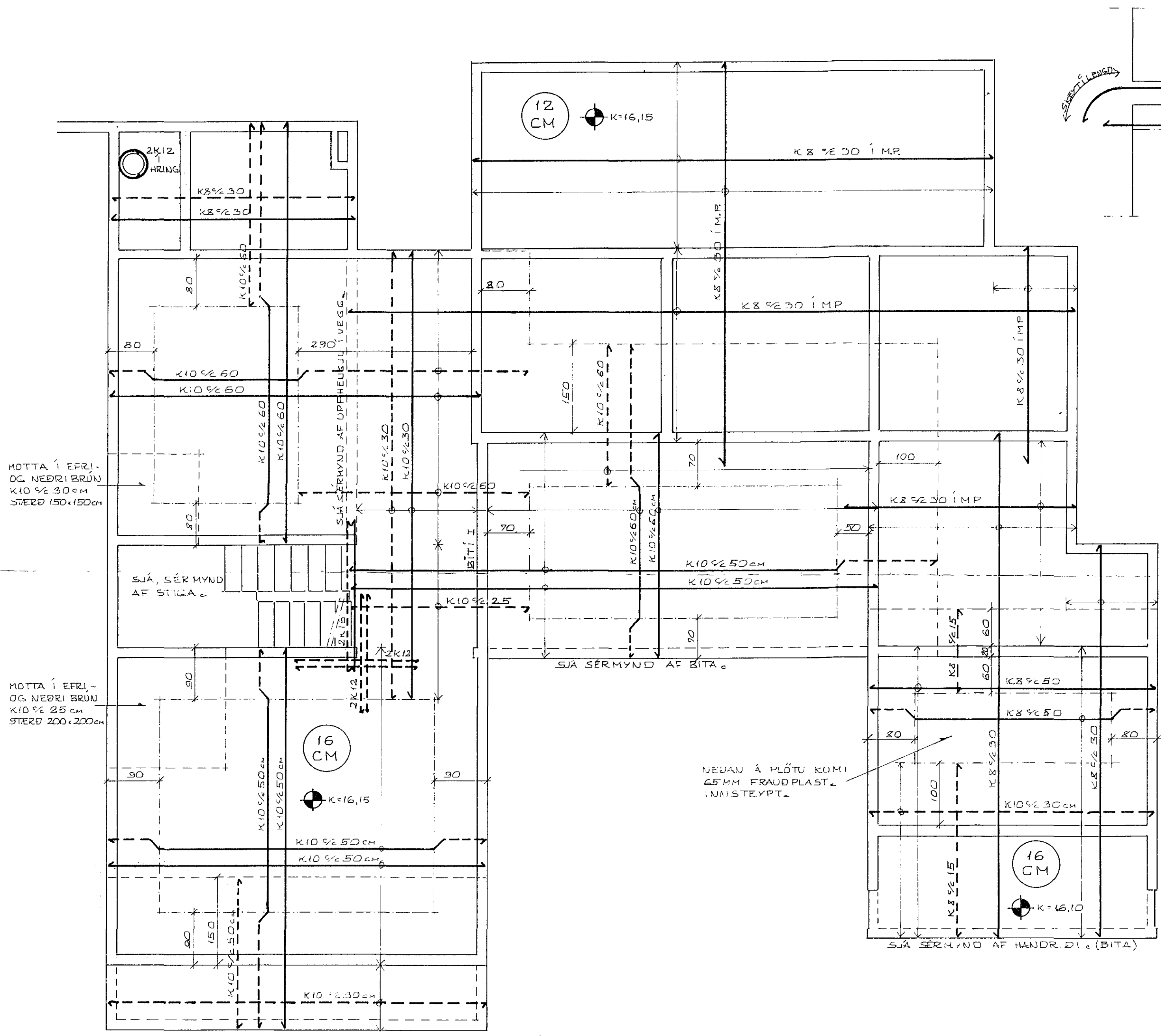
GÓLFPLATA 1. HÆÐAR 1:50
