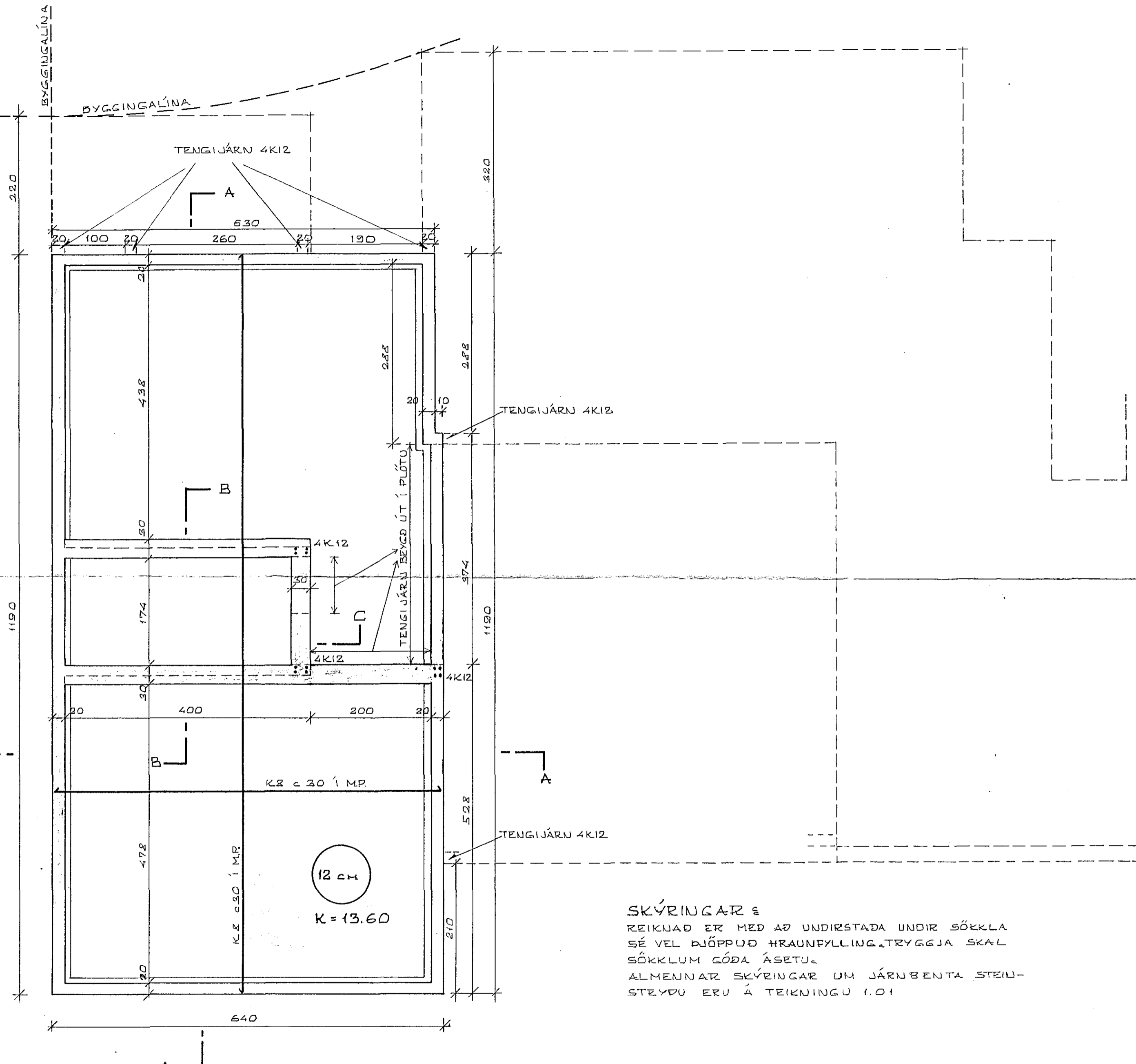
GRUNNMYND 1:50
