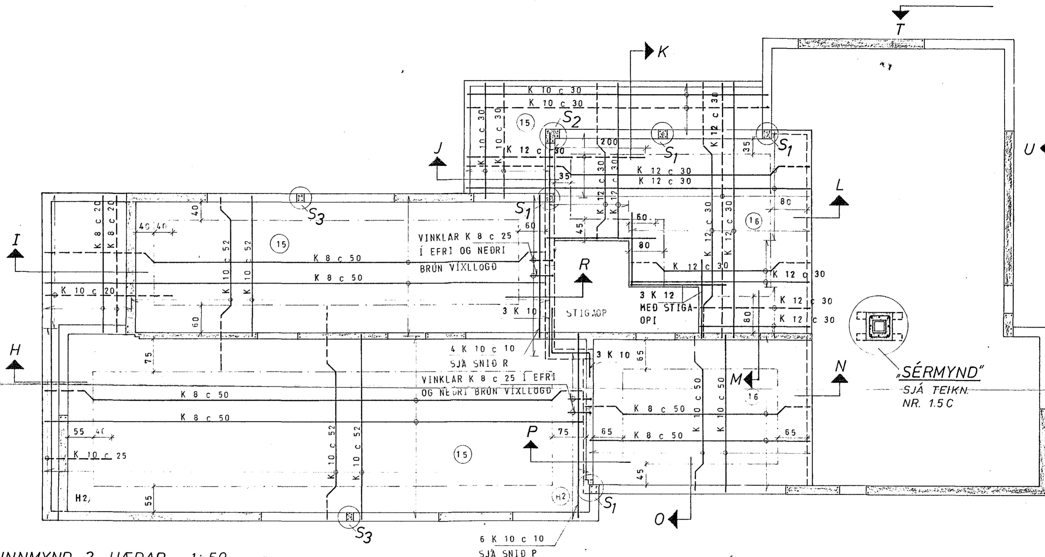
GRUNNMYND 2. HÆÐAR 1:50
