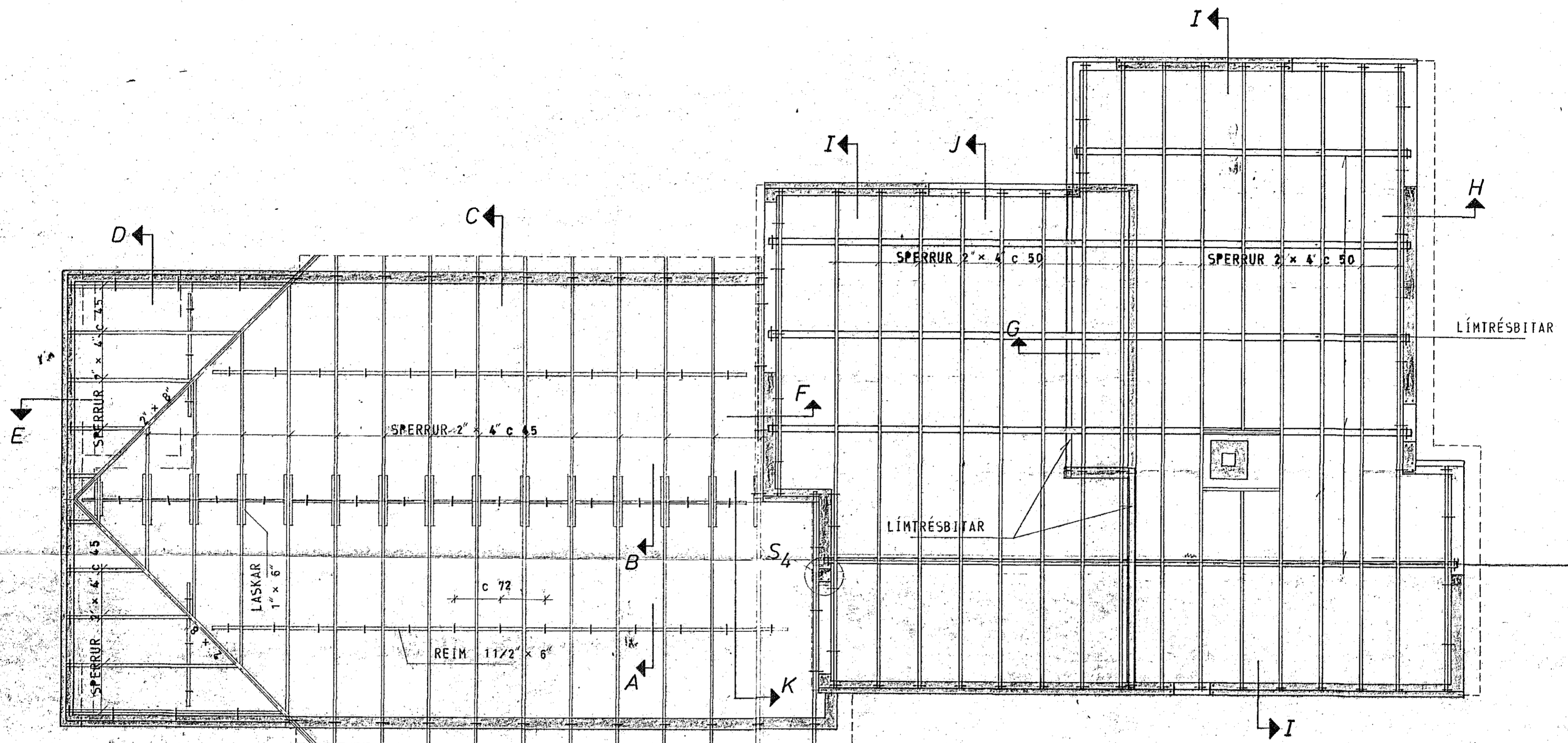
GRUNNMYND PAKS 1:50
