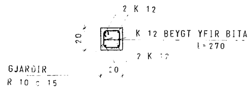
SÚLA S 4 1:20
