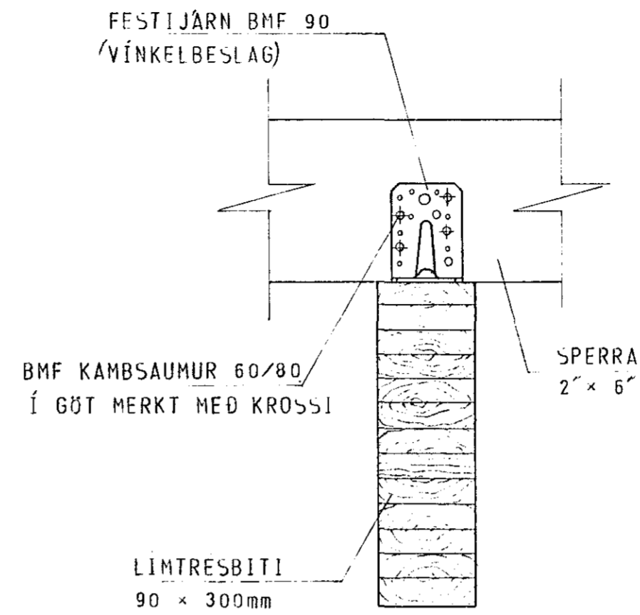
SÉRMYNDIR AF FESTINGUM MILLI SPERRU OG LÍMTRÉSBITA 1:5
