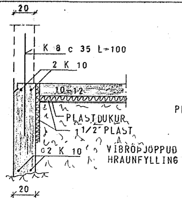
SNÍÐ Í ÚTVEGG 1:20
