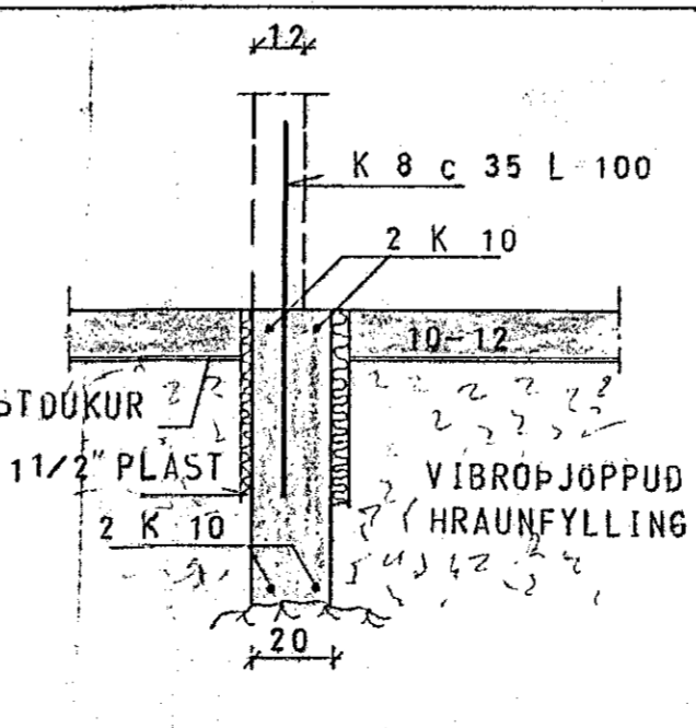
SNÍÐ Í INNVEGG 1:20
