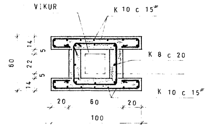
VIKUR AF SKORSTEINI 1:20
