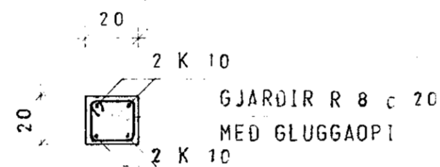
SÚLA S 1 1:20
