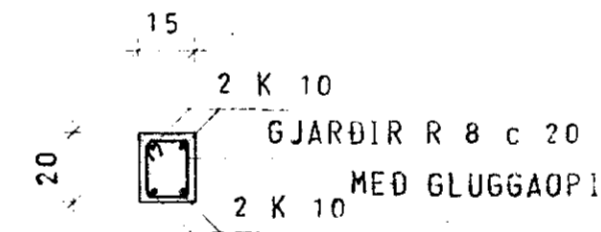
SÚLA S 3 1:20
