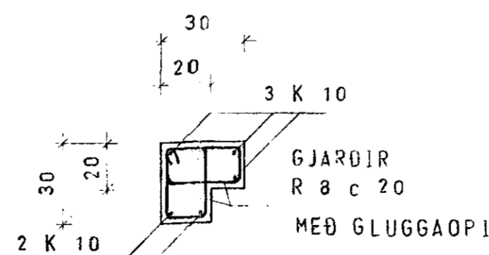
SÚLA S 2 1:20
