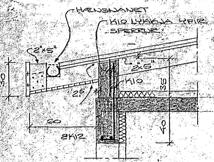
SKURDUR A, M=1:20
