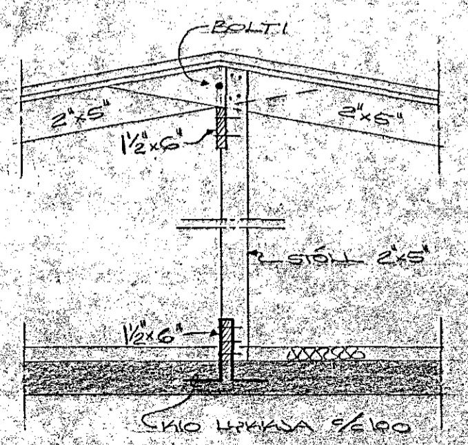
SKURDUR C, M=1:20
