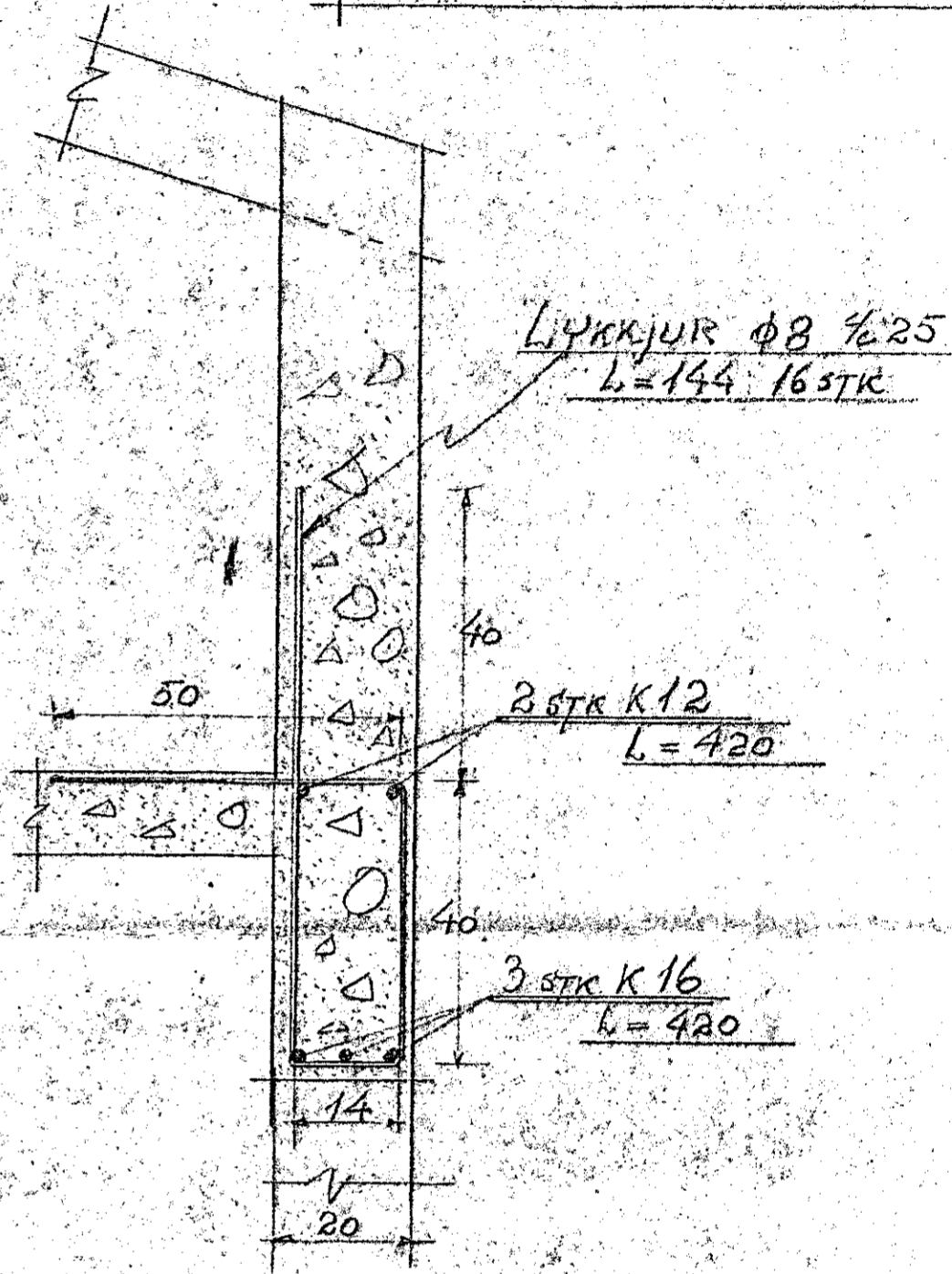
SNIB YFIR GLUGGA Í SJÓNVARPS- OG GARDSTOFU KVARDI 1:10
