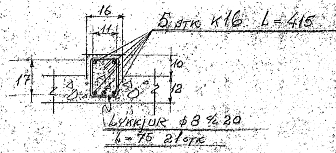
SNIB C-C KVARDI 1:10
