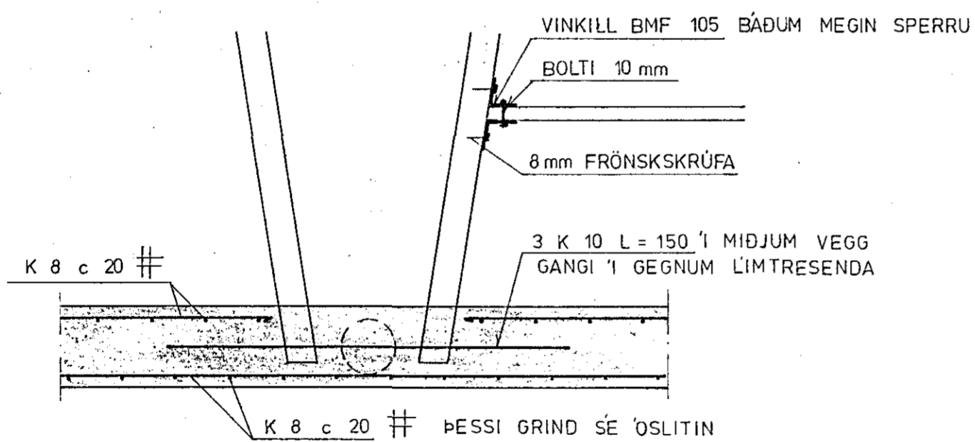
SÉRMYND E 1:20
