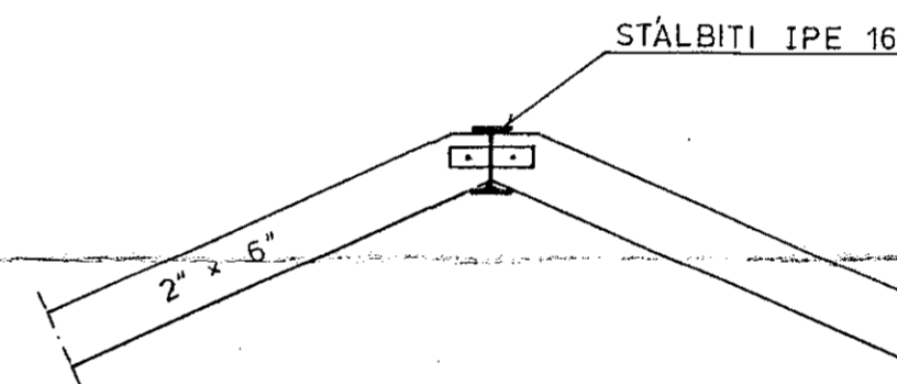
SNID D 1:20
