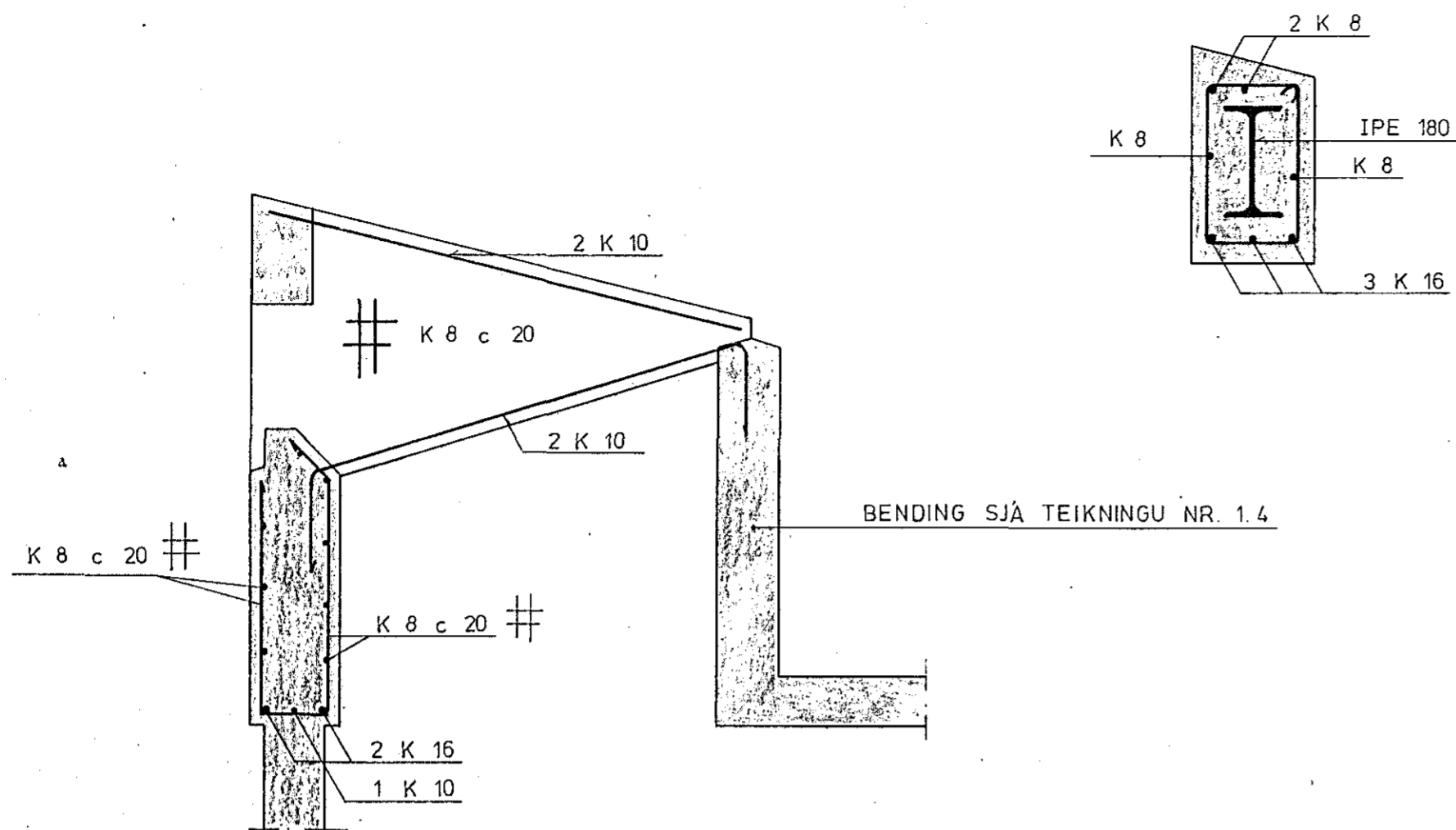
SNID A-A 1:20
