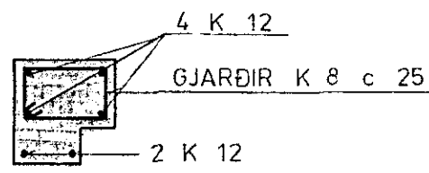
S 1 1 : 20
