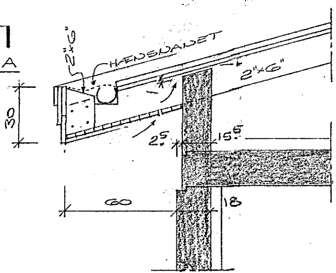
SKURDUR A, M=1:20
