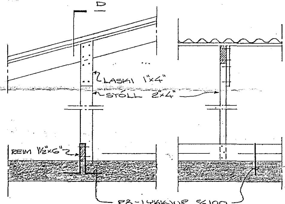
SKURDUR C, M=1:20 SKURDUR D, M=1:20
