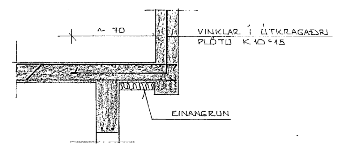
SNID G - G ~ 1:20
