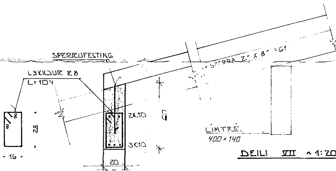
DEILI III \times 1:20
