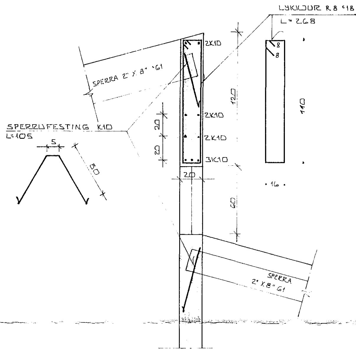
DEILI I \times 1:20
