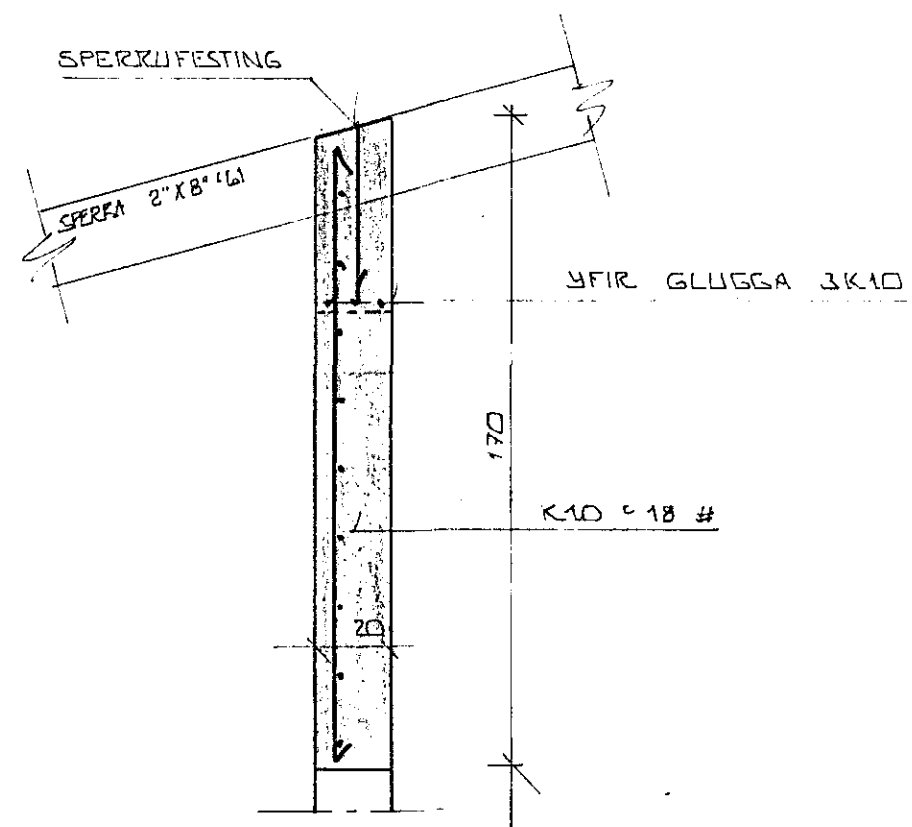
DEILI V \times 1:20
