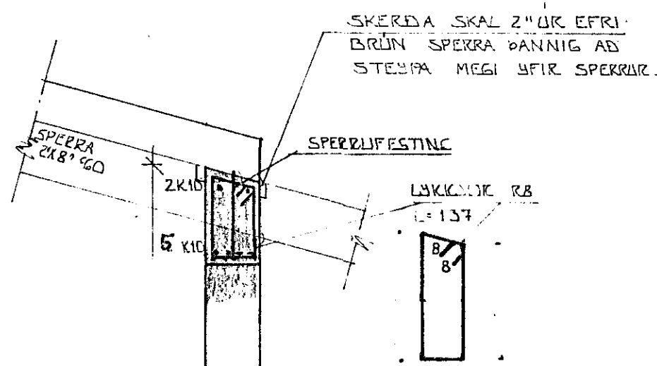
DEILI III \times 1:20
