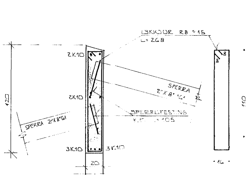
DEILI II \times 1:20
