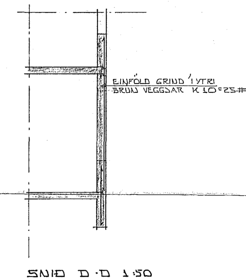
SNID D-D 1:50
