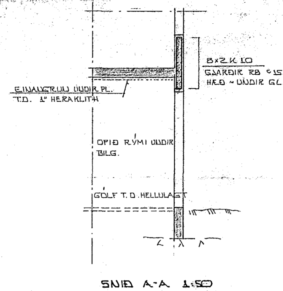
SNID A-A 1:50
