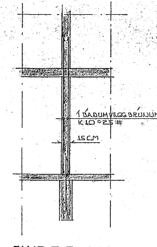
SNID B-B 1:50
