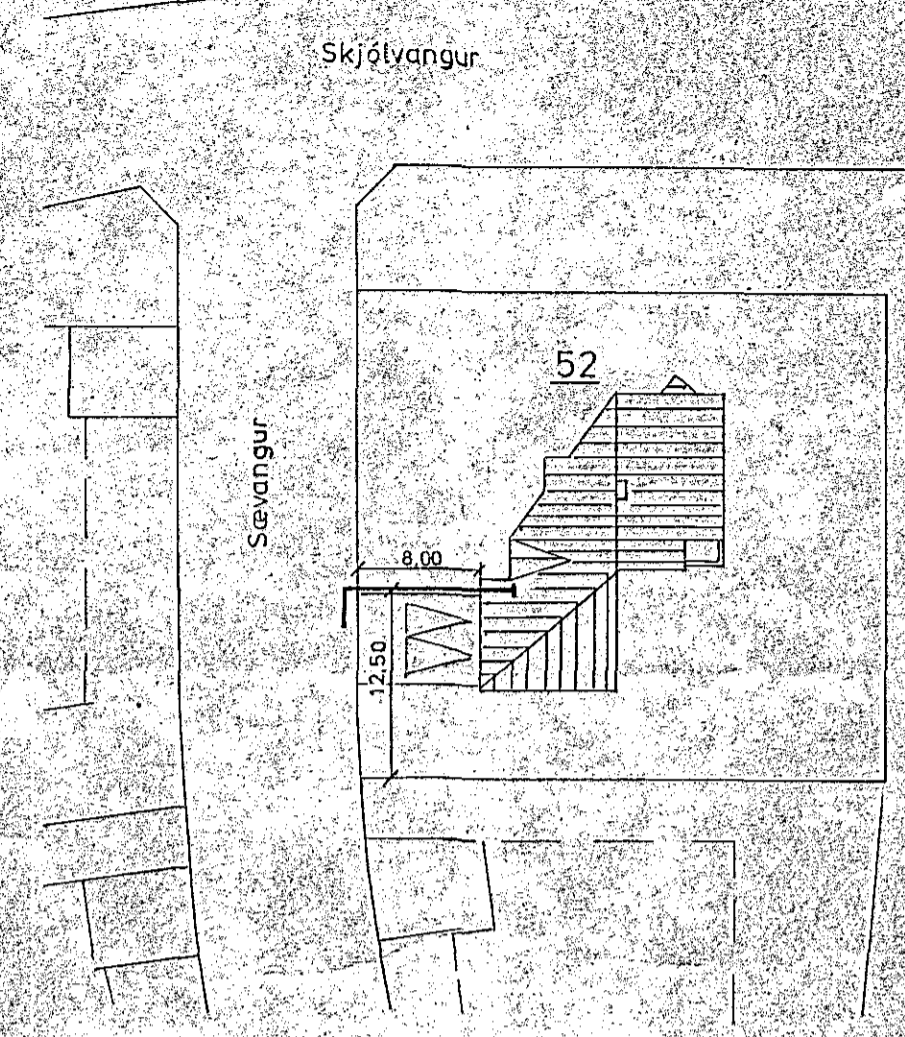
afstöðumynd 1:500
