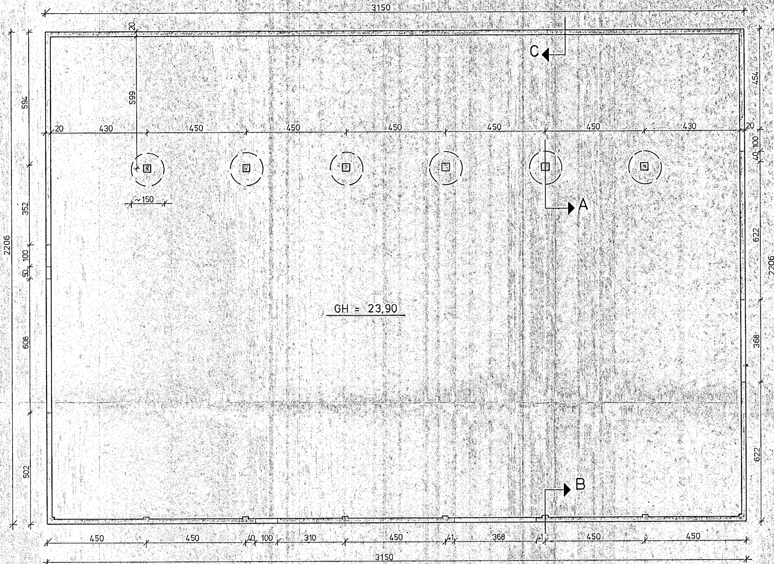
GRUNNMYND 1:100
