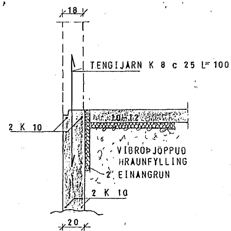
SNID Í ÚTVEGG 1:20
