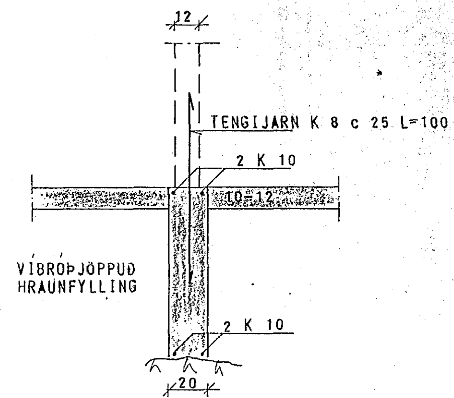
SNID Í INNVEGG 1:20
