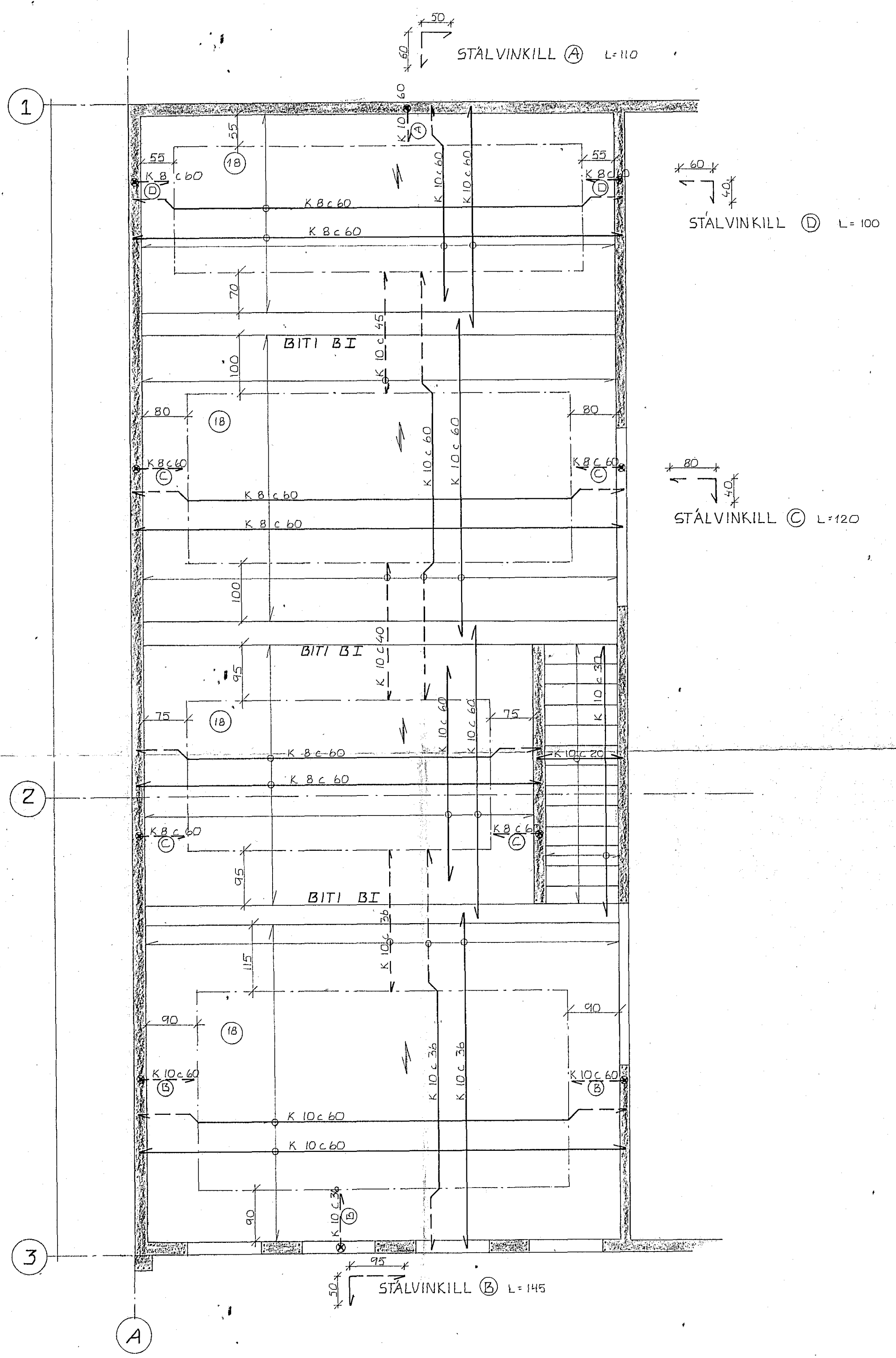
PLATA YFIR JARÐHÆÐ 1:50
