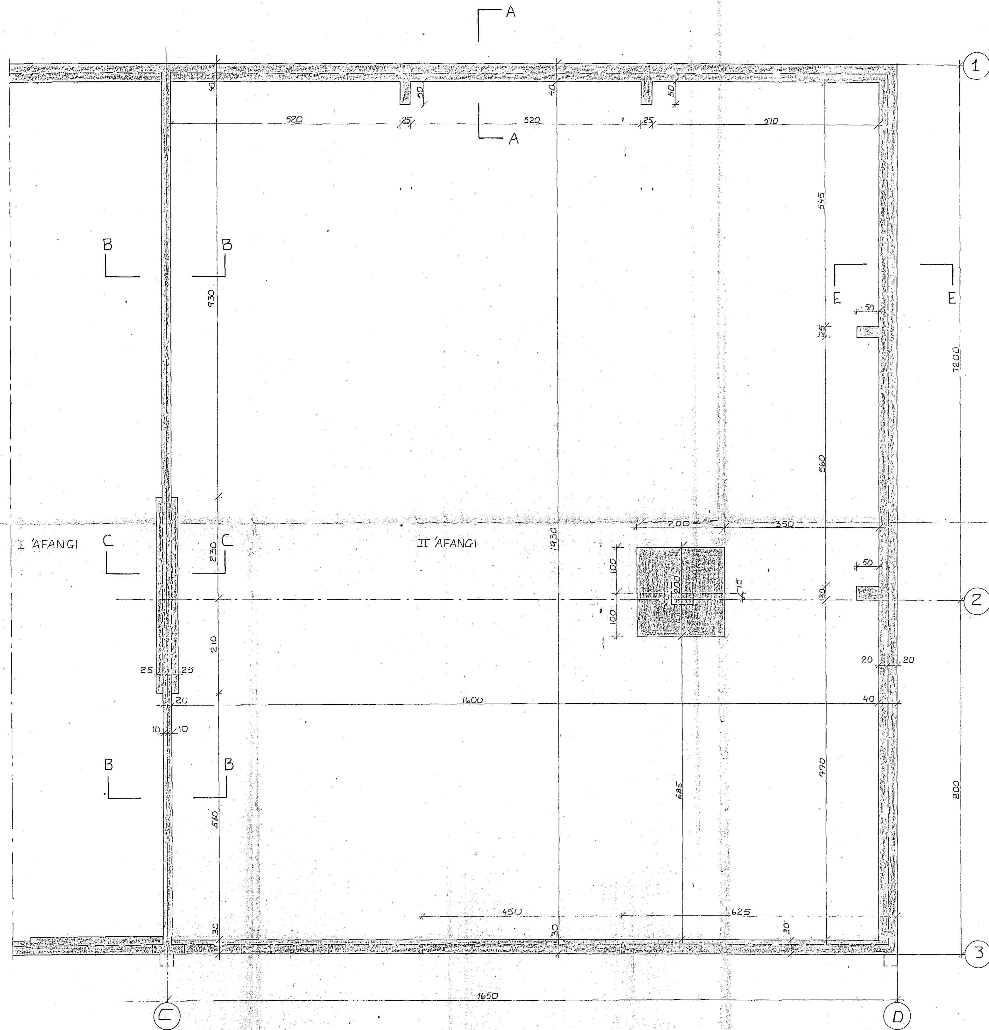
GRUNNMYND 1:50
