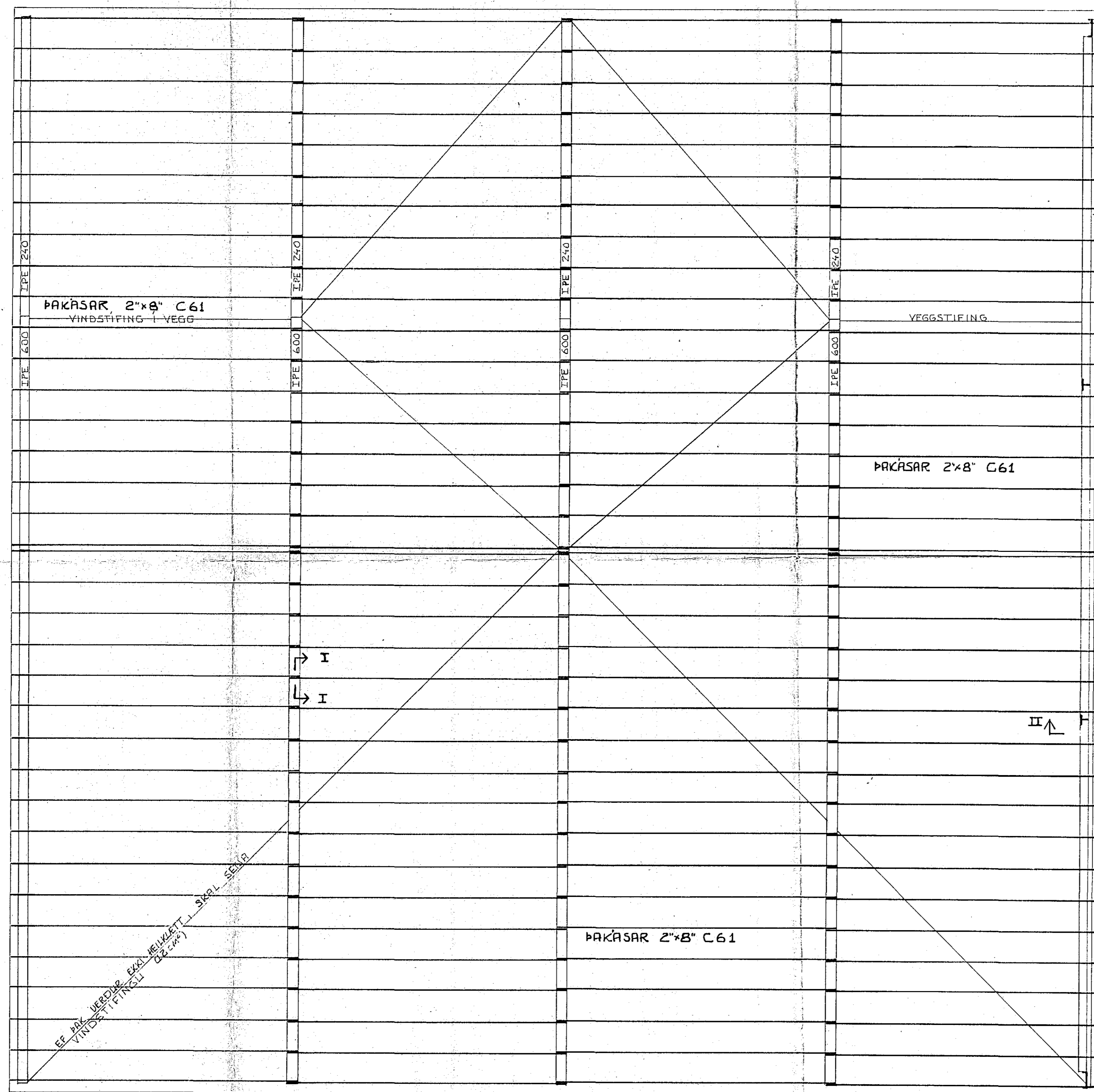
PAKÁSAR GRUNNMYND 1:50
