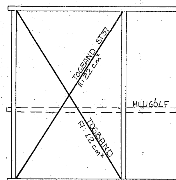
VINDSTIFING Í VEGG 1:100
