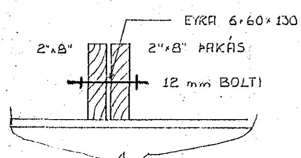
SNID II, FESTING PAKÁSA VIÐ STÁLBITA 1:10
