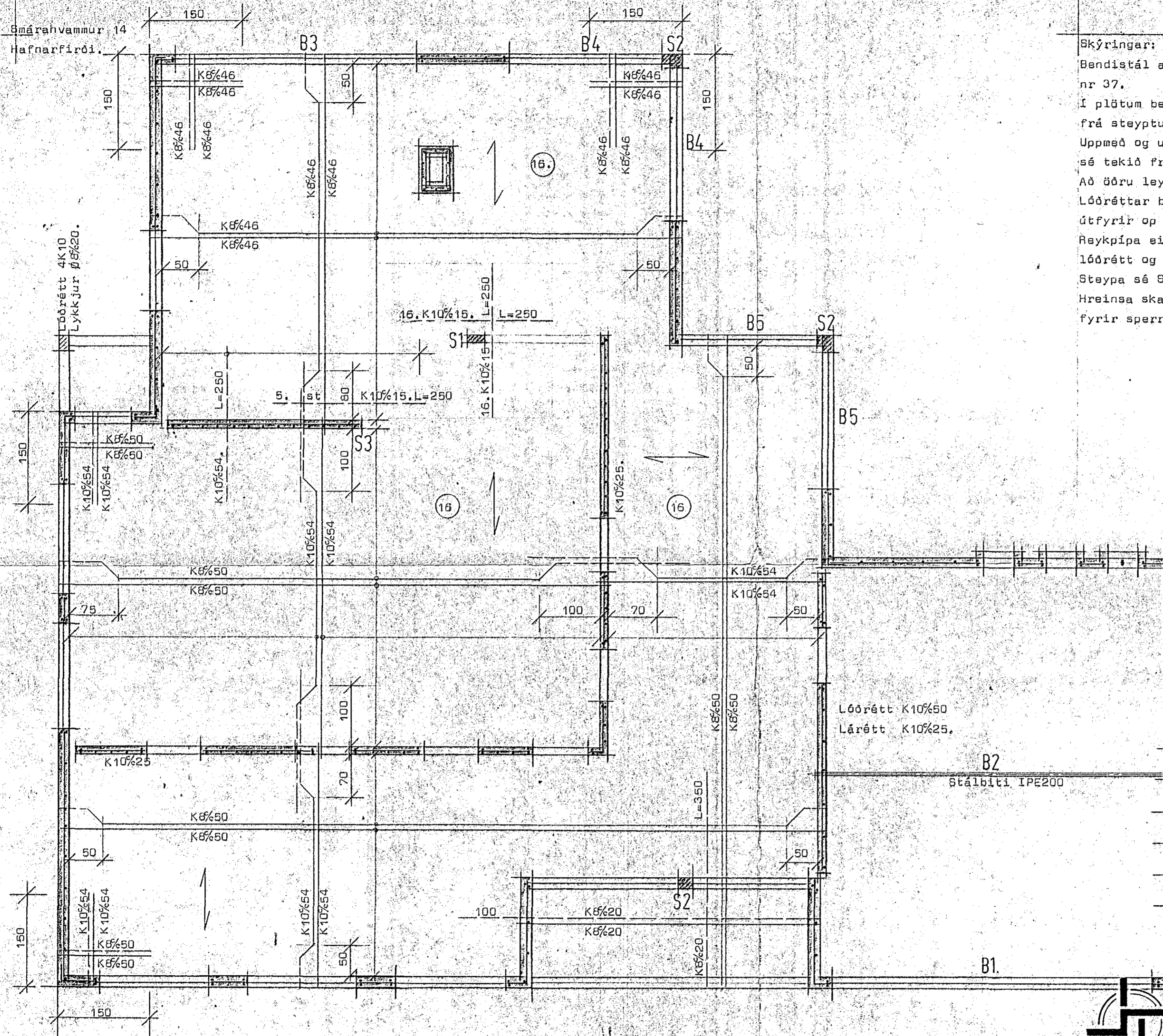
Grunnmynd þakplötu mk 1:50
