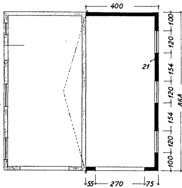
Grunnmynd
