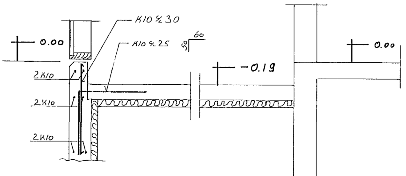
SNID A-A HÚS NR 62
