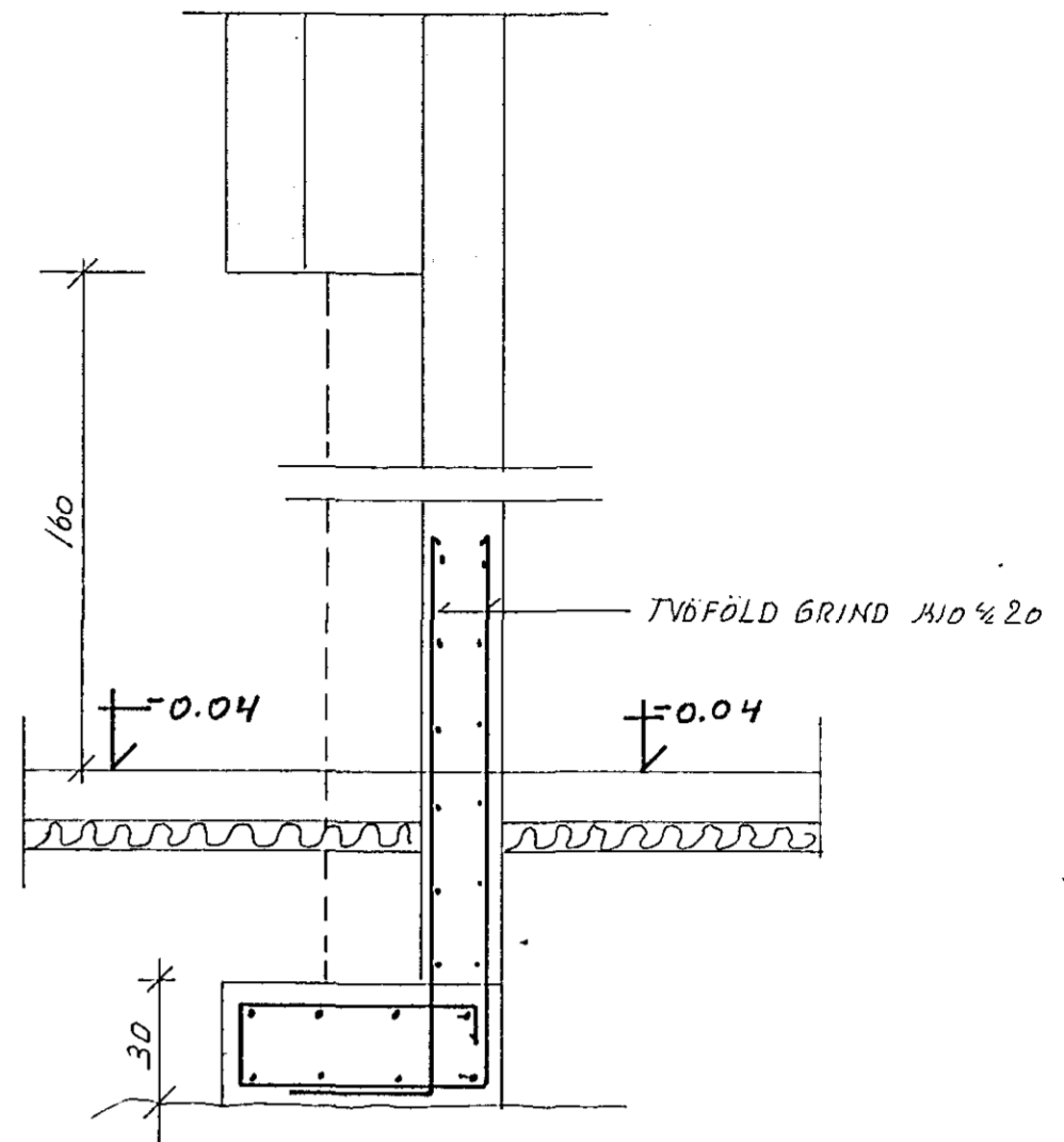
SNID B-B HÚS NR 60
