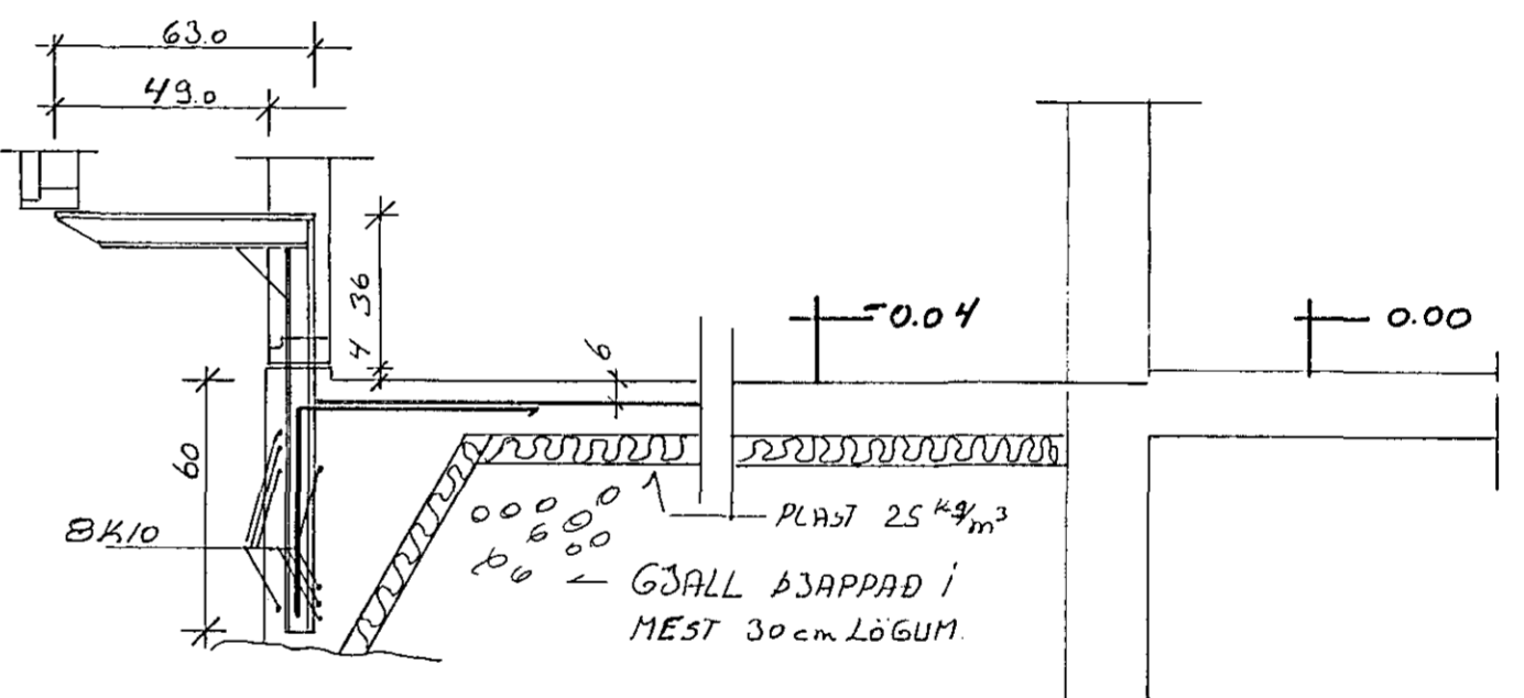
SNID A-A HÚS NR 60 06 52
