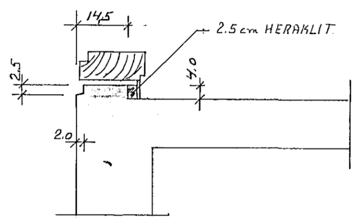
FRÁGANGUR UNDIR GLUGGA 1:10
