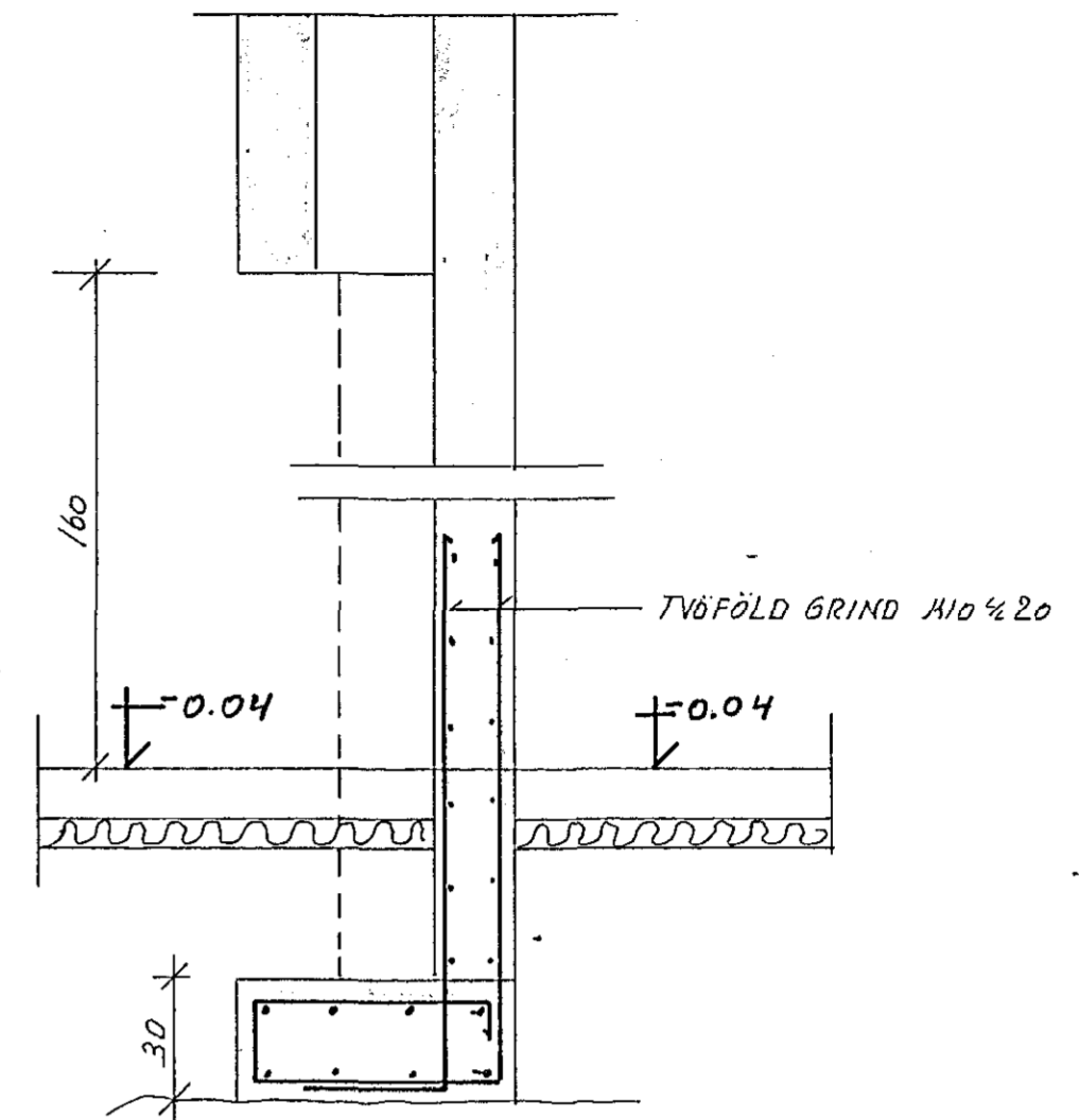
SNID B-B HÚS NR 60
