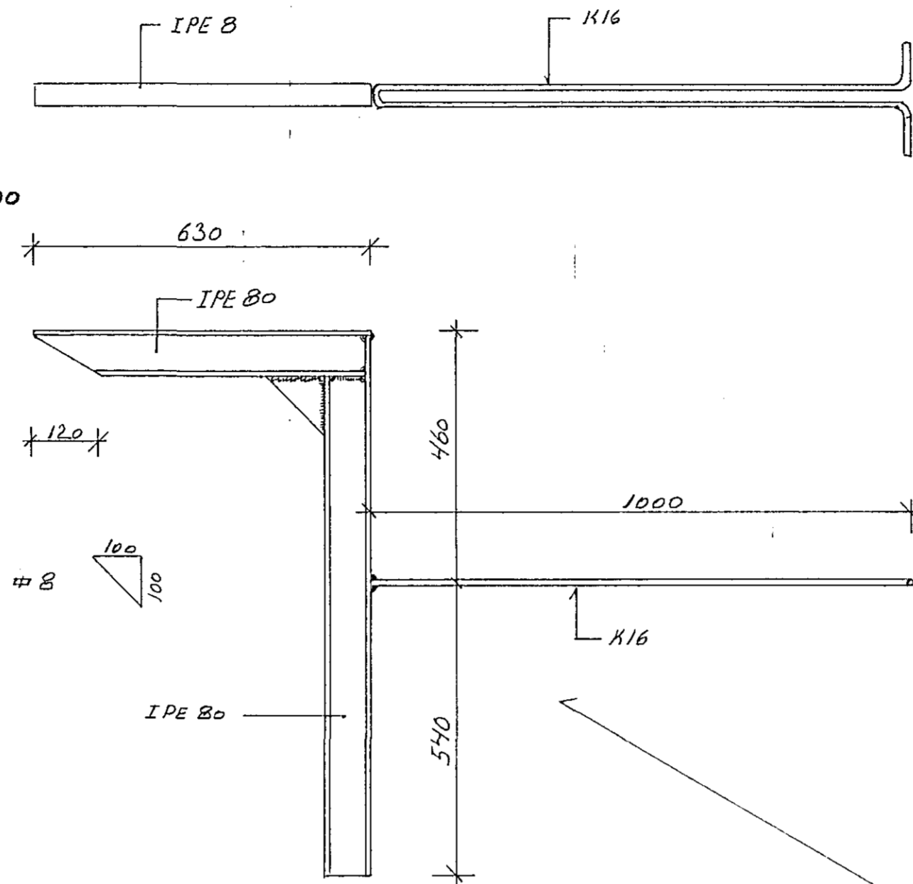
FESTING UNDIR GLUGGA Í HÚSUM NR 54 06 60 2 STK Í HVORU HÚSI.
