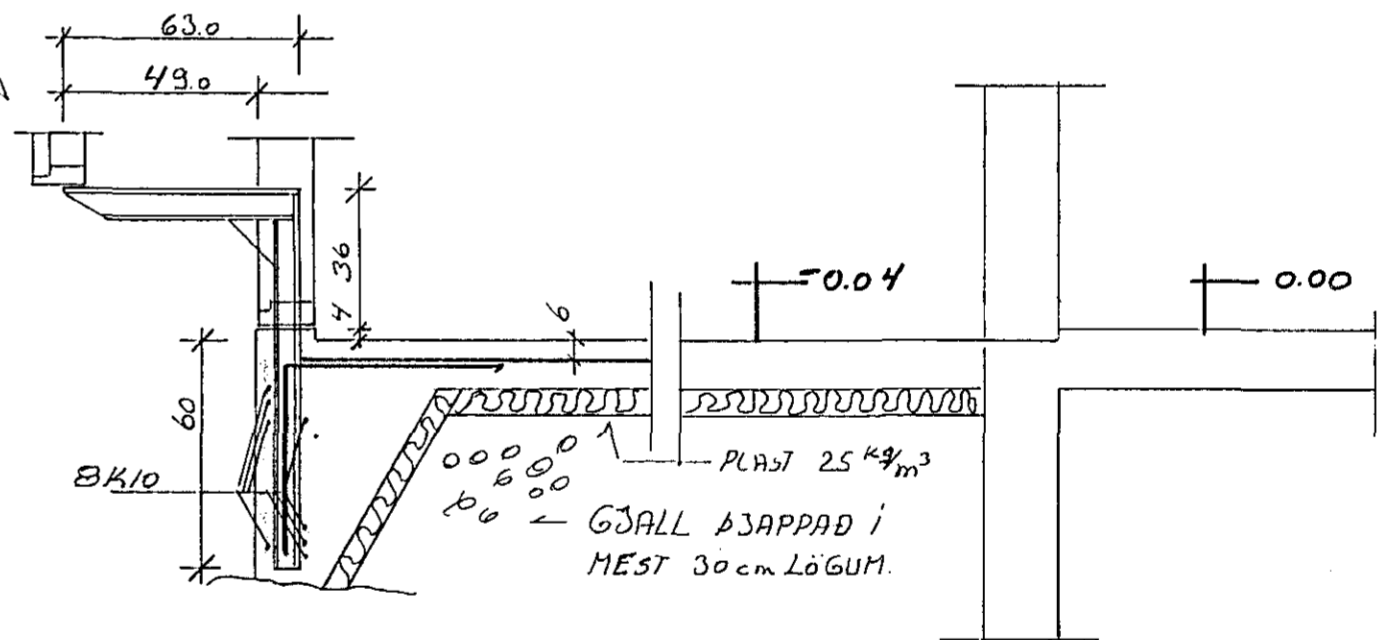
SNID A-A HÚS NR 60 06 52
