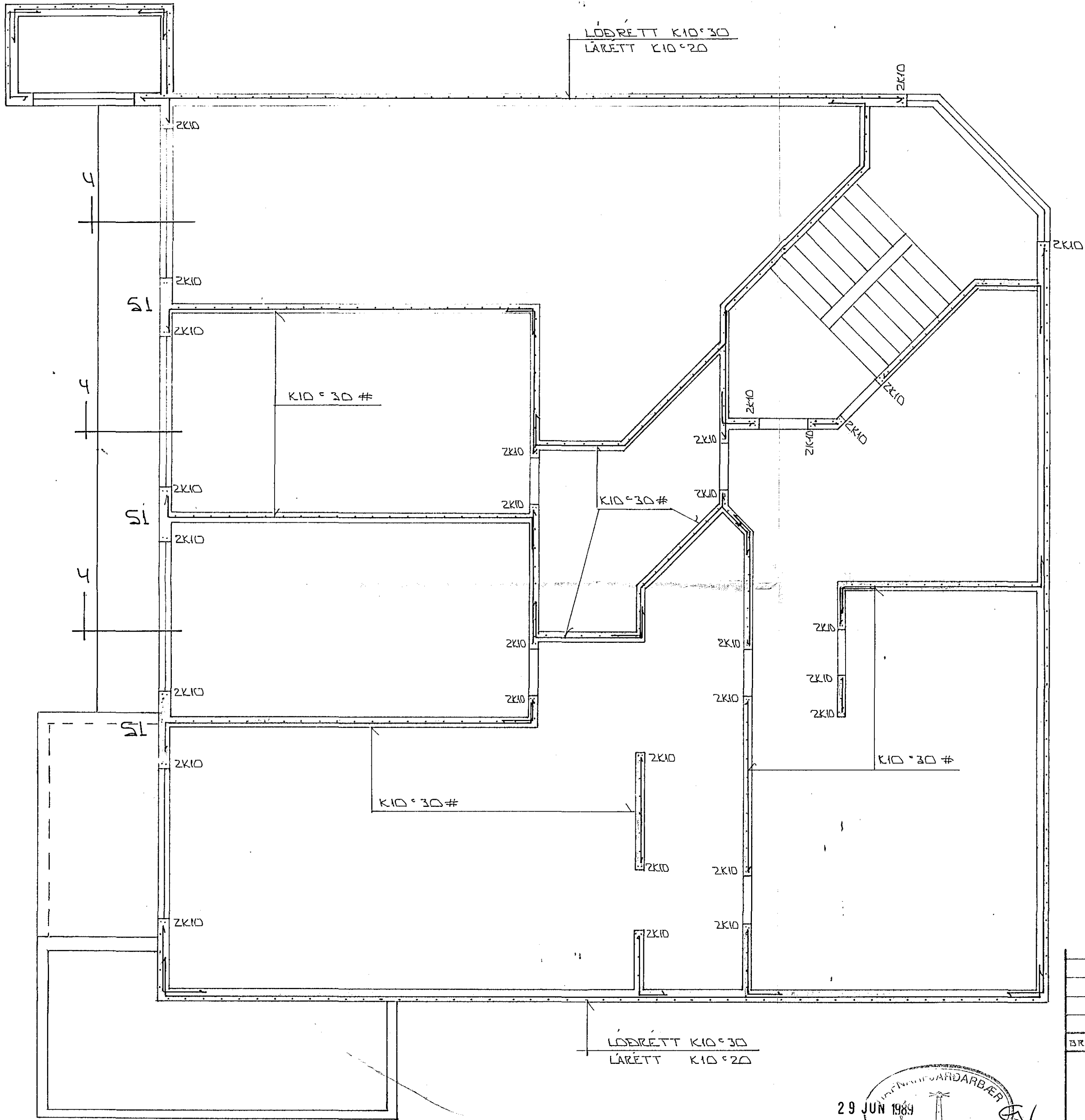
GRUNNMYND KJALLARA 1:50
