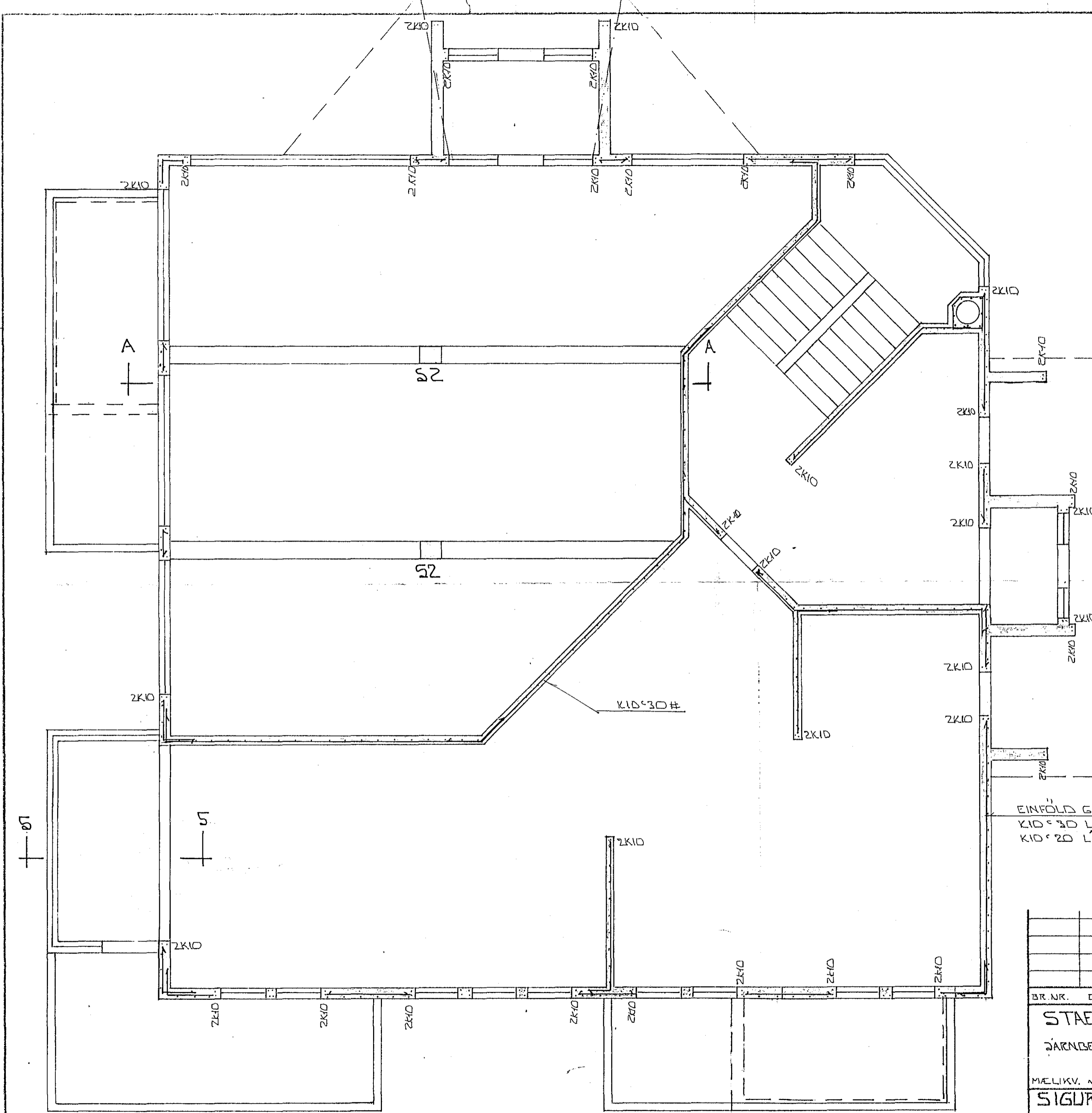
GRUNNMYND 1. HÆÐ 1:50
